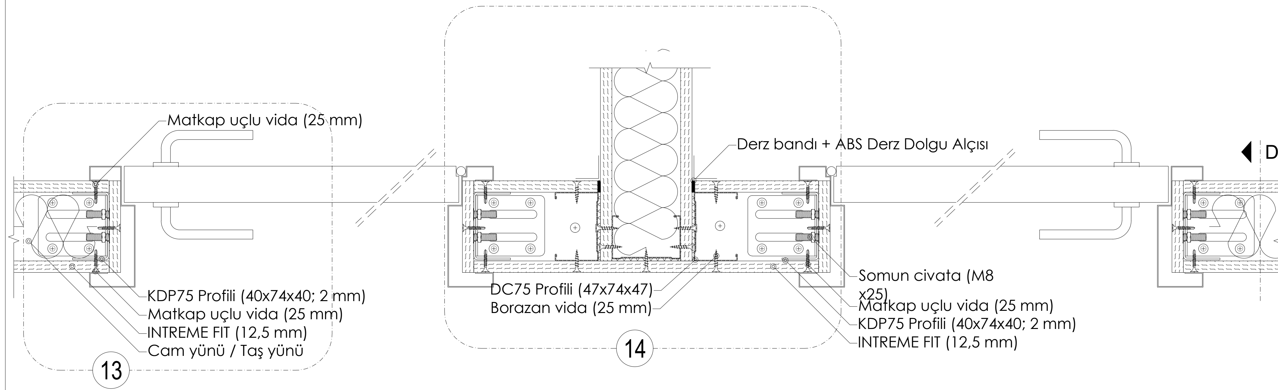
PLAN: TEK İSKELET SİSTEMİ KAPI DESTEK PROFİLİ DETAYI
