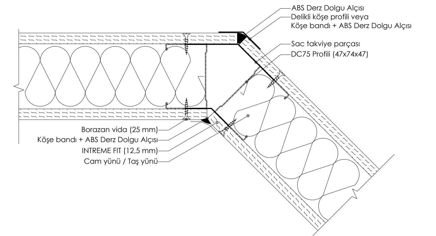
DETAY 08: TEK İSKELET SİSTEMİ 135° DUVAR BİRLEŞİMİ
