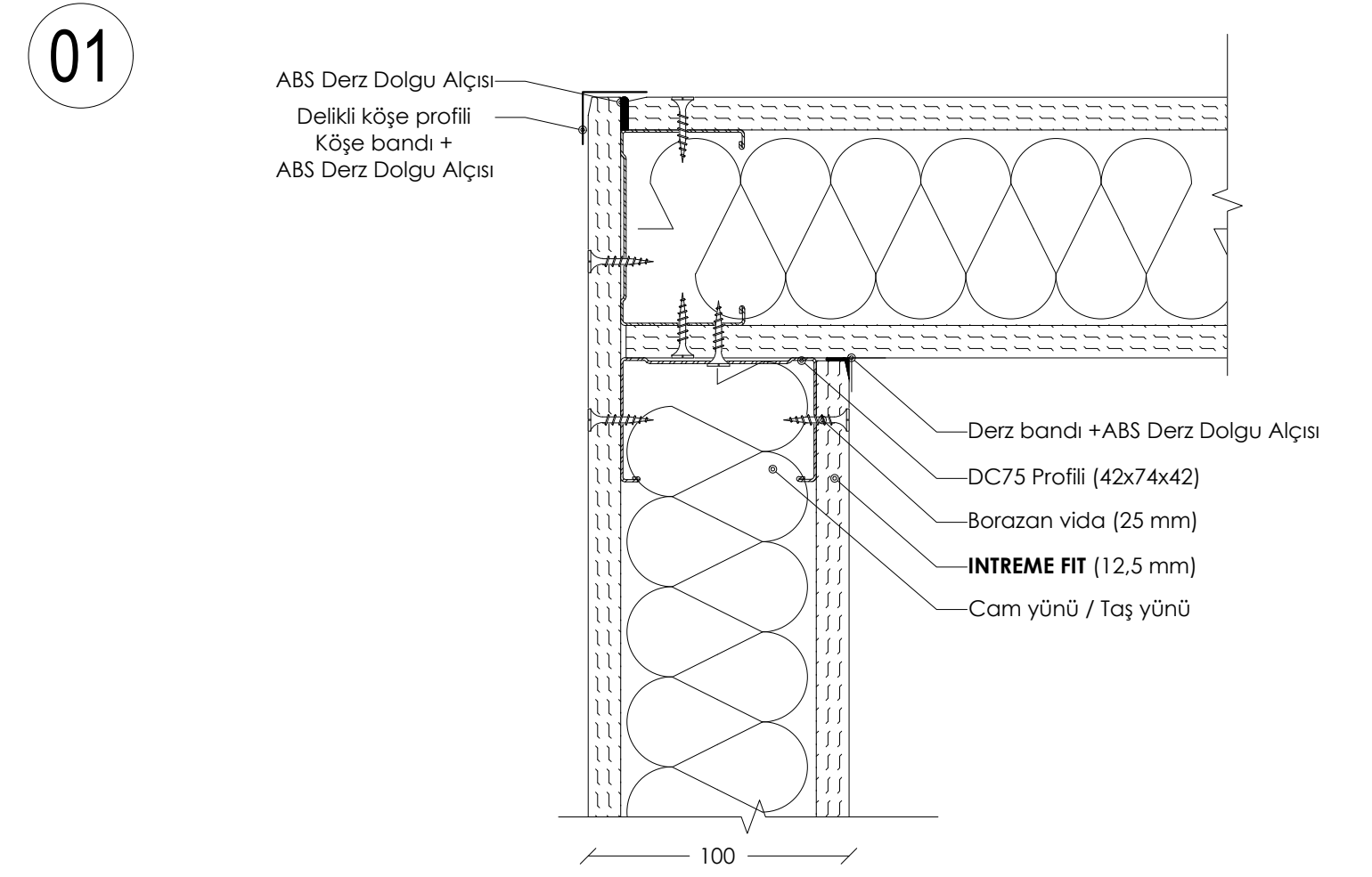
DETAY 01: TEK İSKELET SİSTEMİ KÖŞE BİRLEŞİM PLANI
