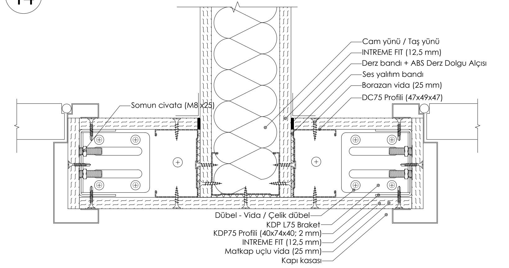
DETAY 14: TEK İSKELET SİSTEMİ KAPI DESTEK PROFİLİ DETAYI
