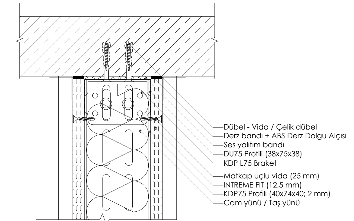
DETAY 16: TEK İSKELET SİSTEMİ KAPI DESTEK PROFİLİ TAVAN BİRLEŞİM KESİTİ
