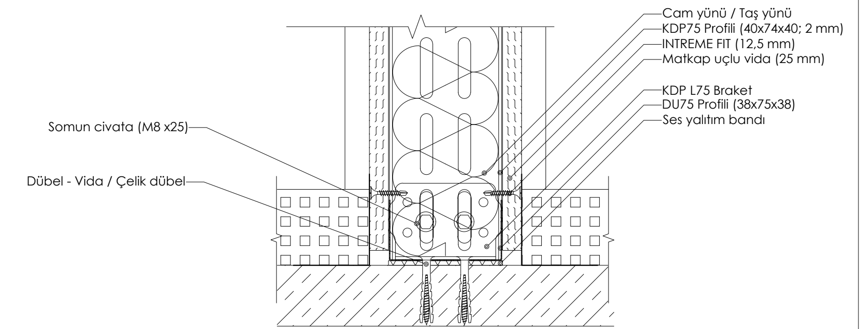
DETAY 15: TEK İSKELET SİSTEMİ KAPI DESTEK PROFİLİ ZEMİN BİRLEŞİM KESİTİ
