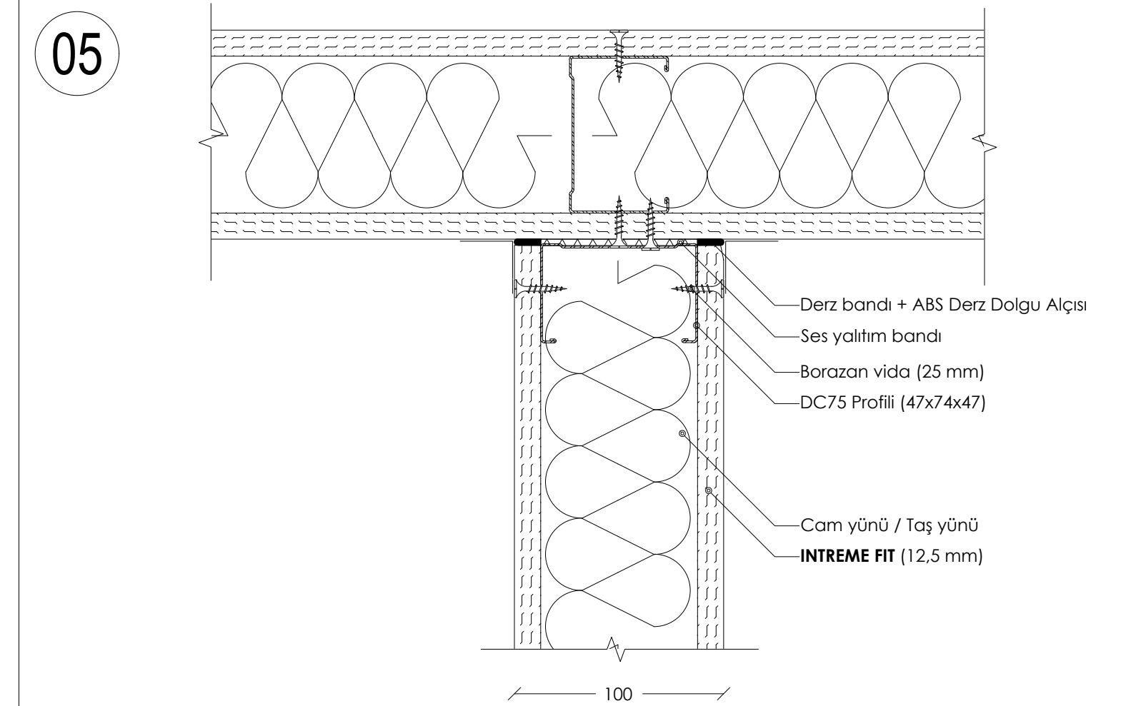
DETAY 05: TEK İSKELET SİSTEMİ BİRLEŞİM PLANI
