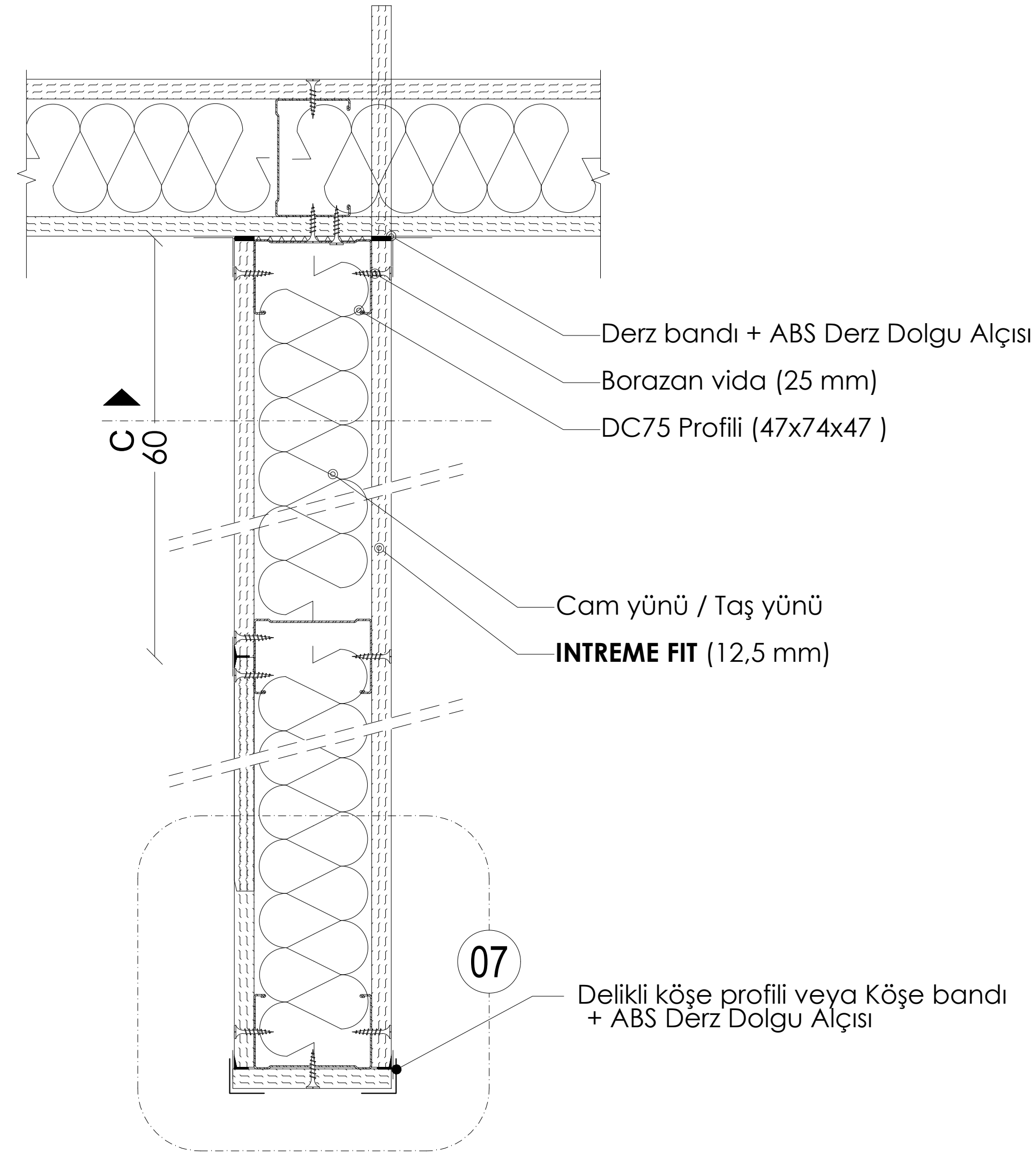
PLAN: TEK İSKELET SİSTEMİ DIŞ DUVAR
