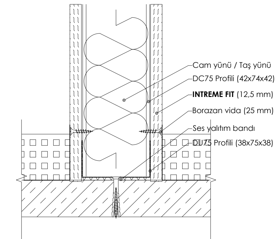
DETAY 04: TEK İSKELET SİSTEMİ ZEMİN BİRLEŞİM KESİTİ
