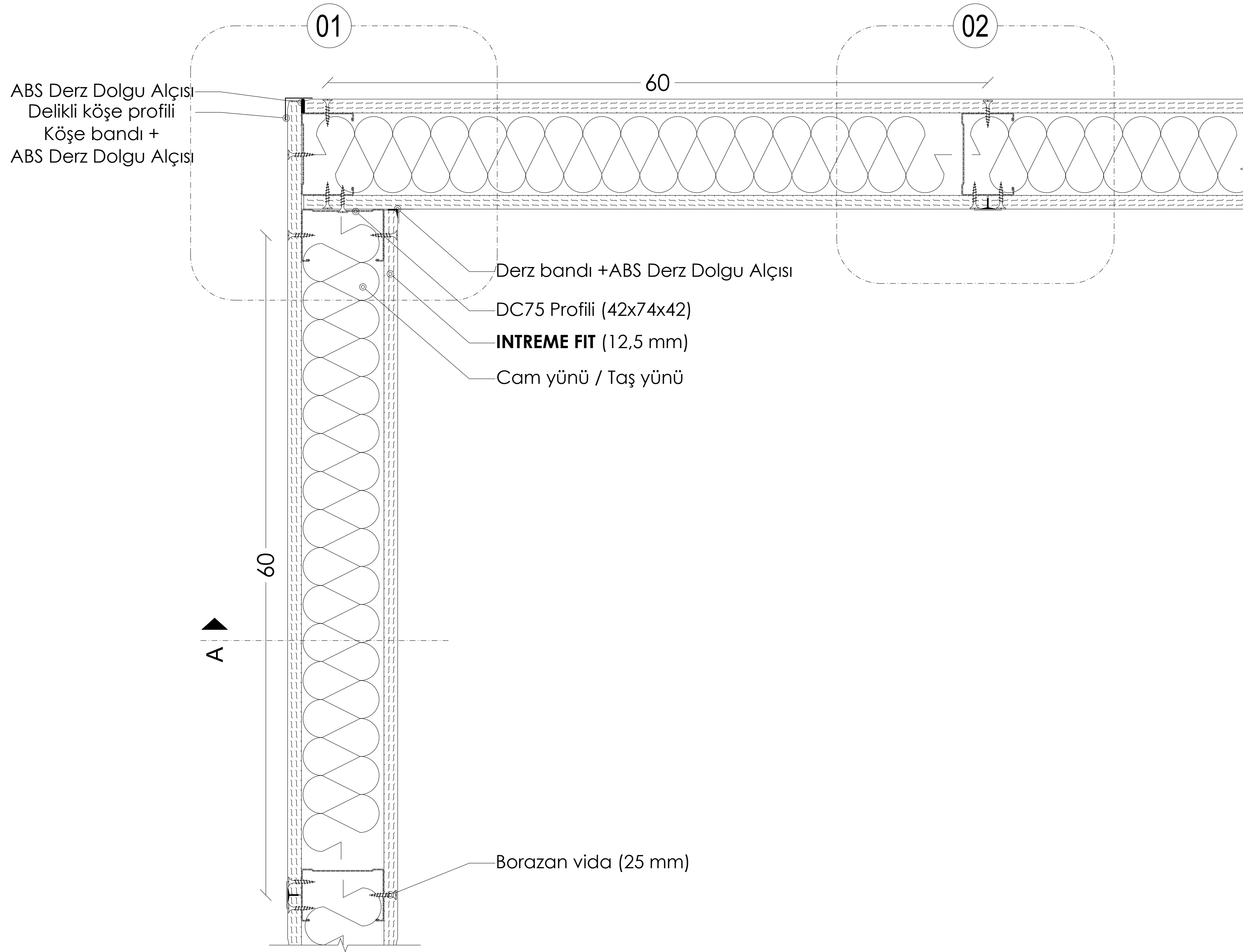
PLAN : TEK İSKELET SİSTEMİ KÖŞE BİRLEŞİMİ
