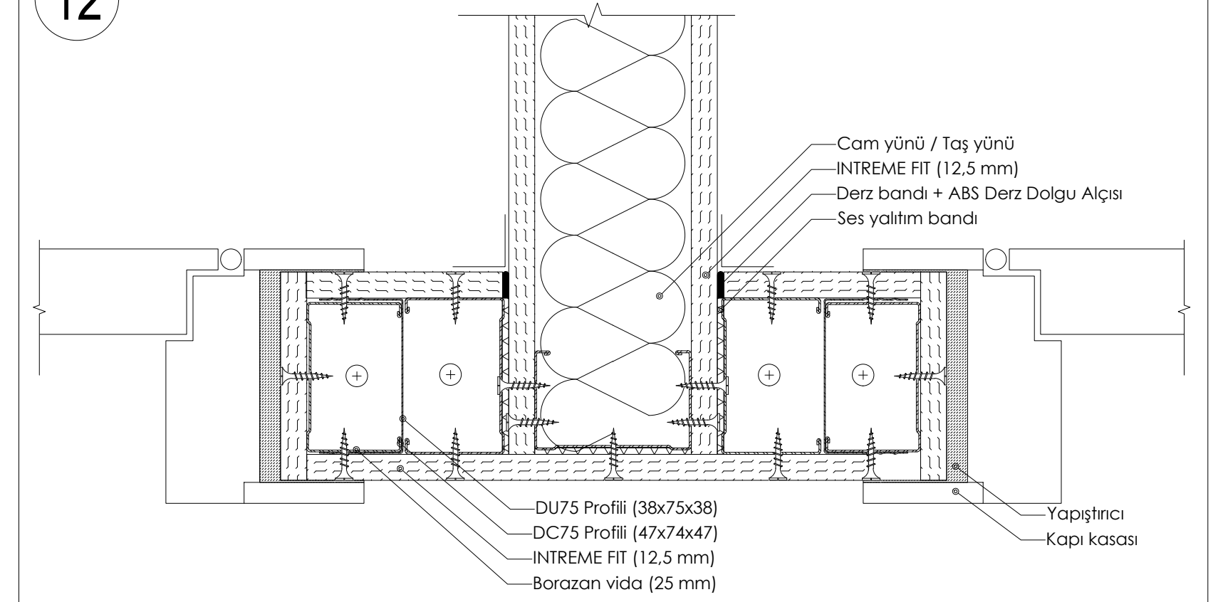
DETAY 12: TEK İSKELET SİSTEMİ KAPI PLANI (YAPIŞTIRMA)
