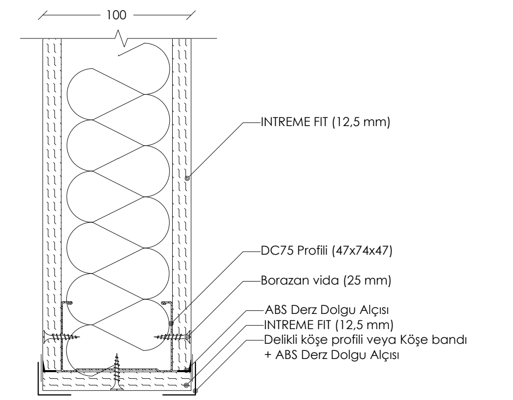
DETAY 05: TEK İSKELET SİSTEMİ BİRLEŞİM PLANI
