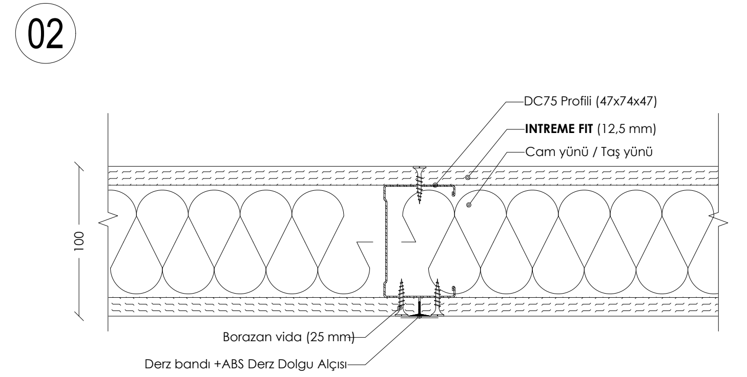
DETAY 02: TEK İSKELET SİSTEMİ BİRLEŞİM PLANI
