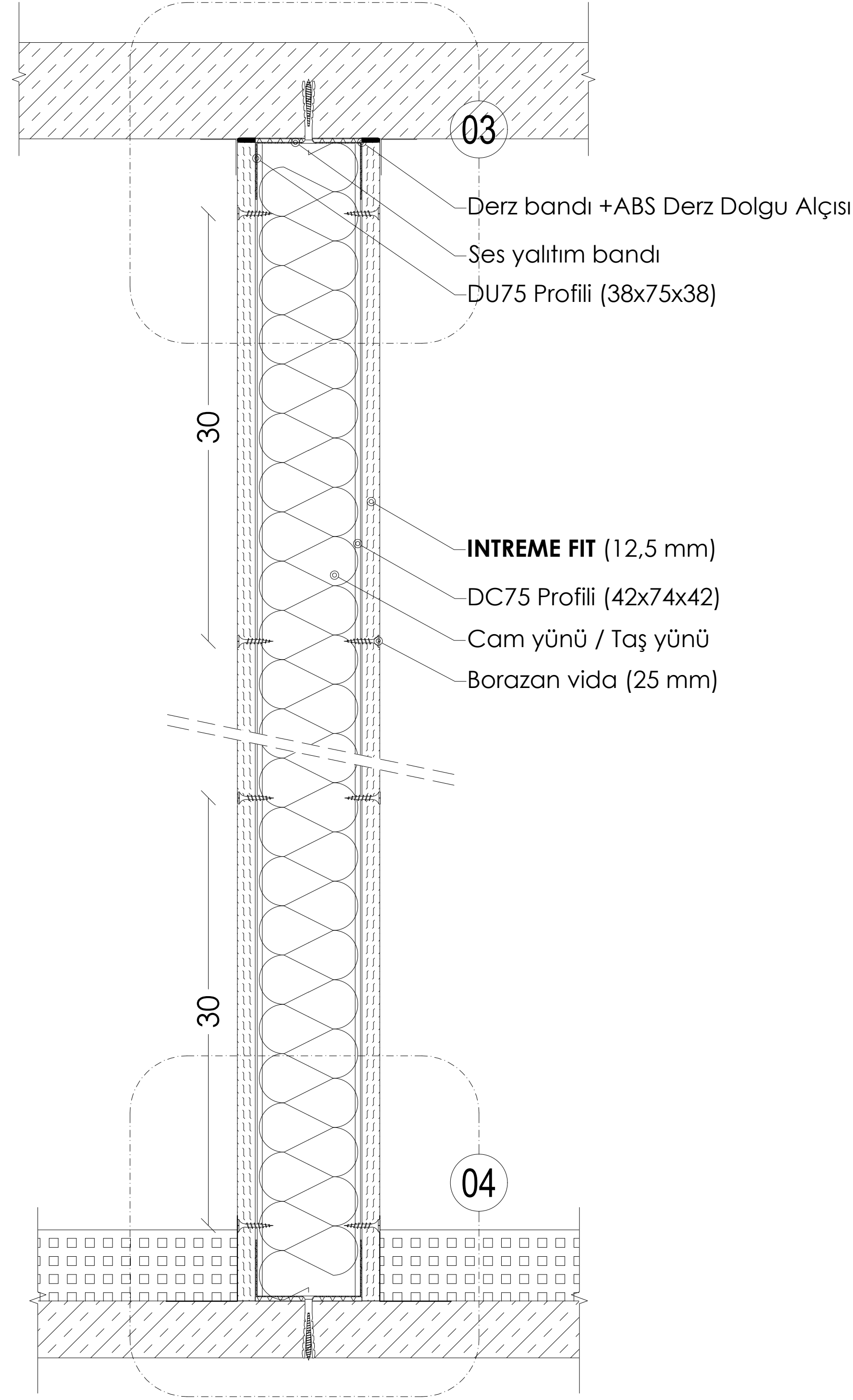
KESİT A: TEK İSKELET SİSTEMİ
