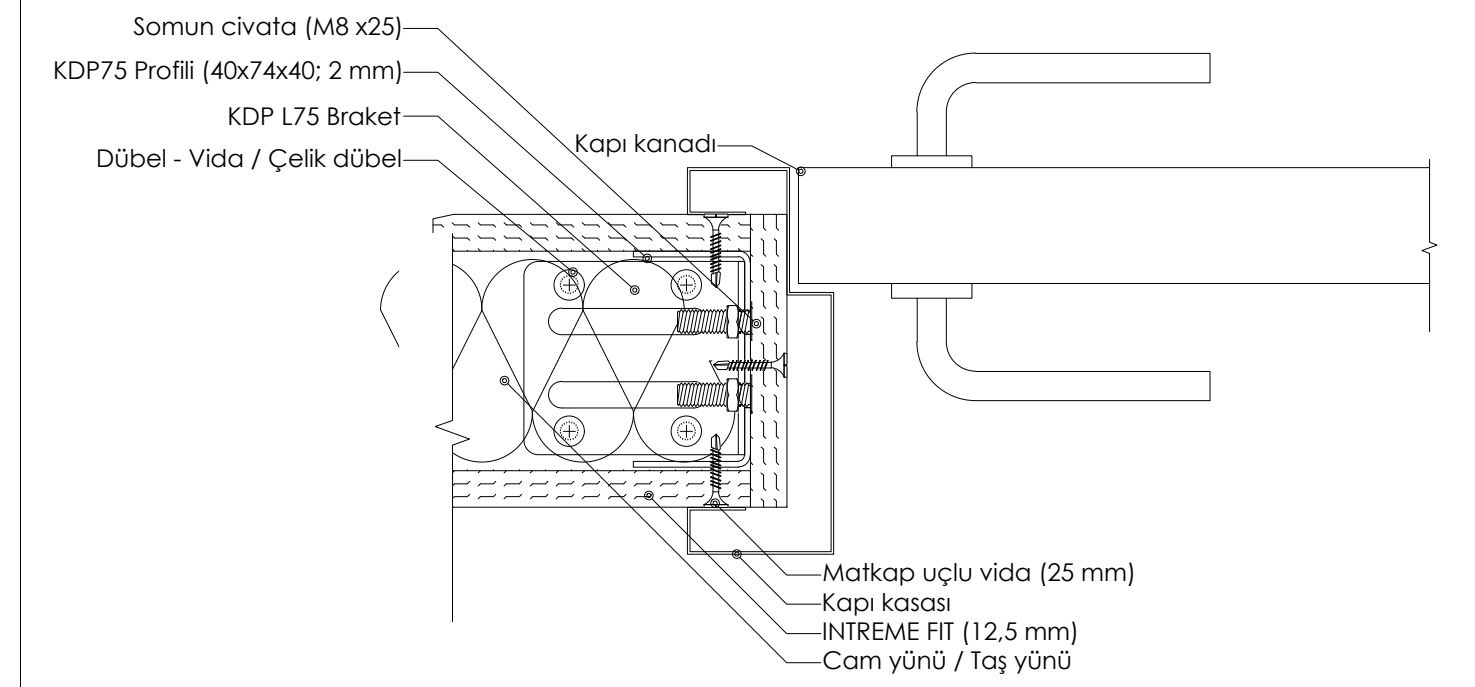
DETAY 13: TEK İSKELET SİSTEMİ KAPI DESTEK PROFİLİ DETAYI
