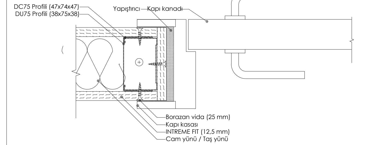
DETAY 11: TEK İSKELET SİSTEMİ KAPI PLANI (YAPIŞTIRMA)
