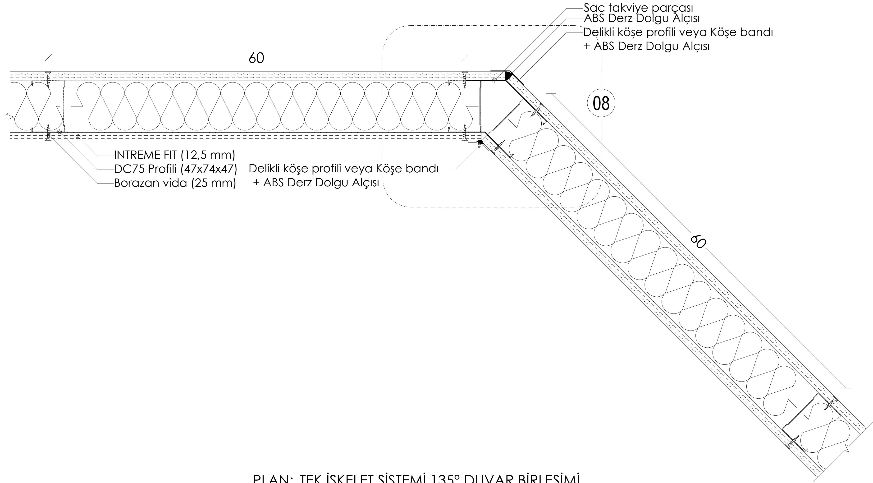
PLAN: TEK İSKELET SİSTEMİ 135° DUVAR BİRLEŞİMİ
