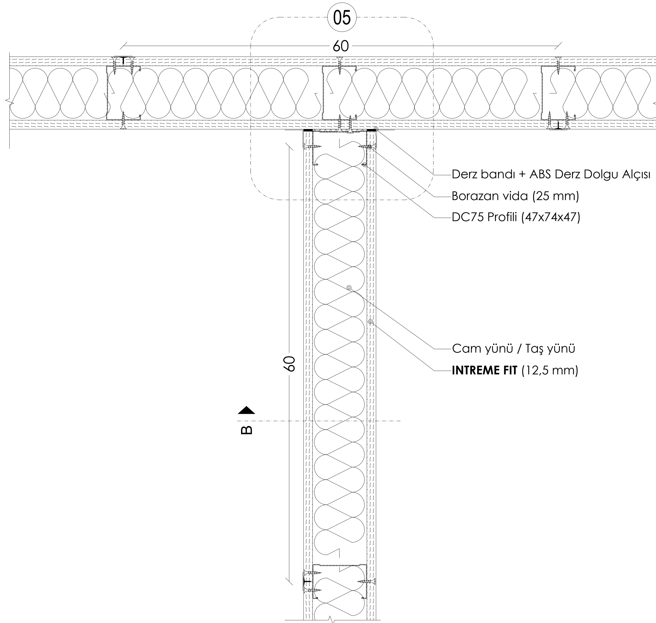
PLAN: TEK İSKELET SİSTEMİ KÖŞE BİRLEŞİMİ
