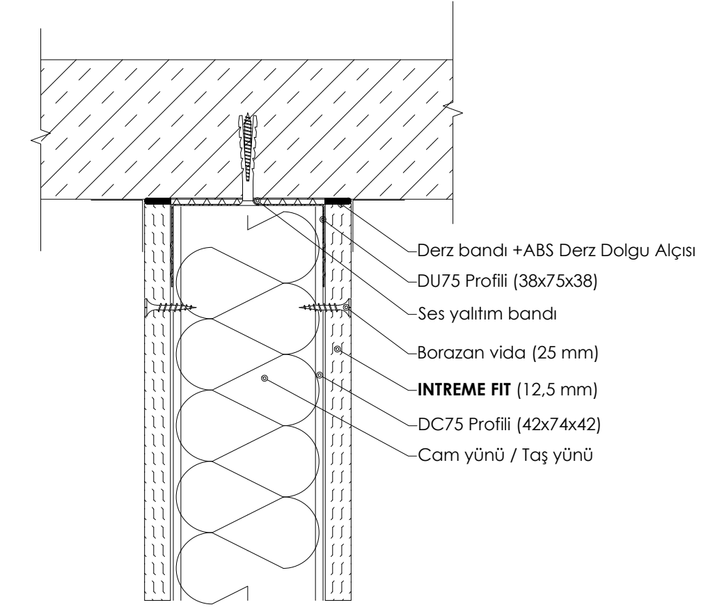
DETAY 03: TEK İSKELET SİSTEMİ TAVAN BİRLEŞİM KESİTİ
