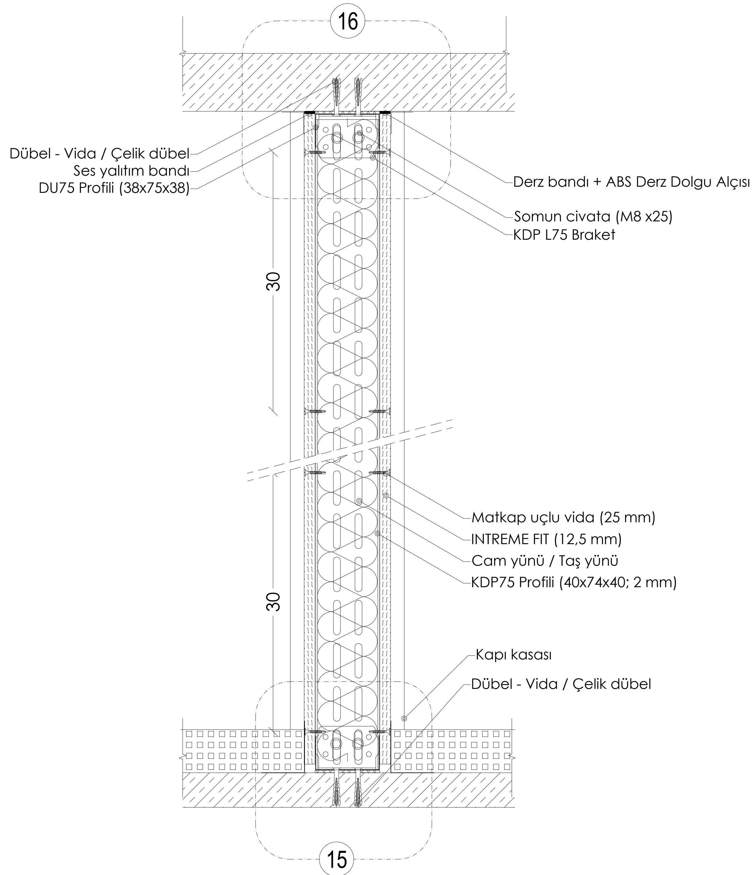
KESİT D: TEK İSKELET SİSTEMİ KAPI DESTEK PROFİLİ DETAYI
