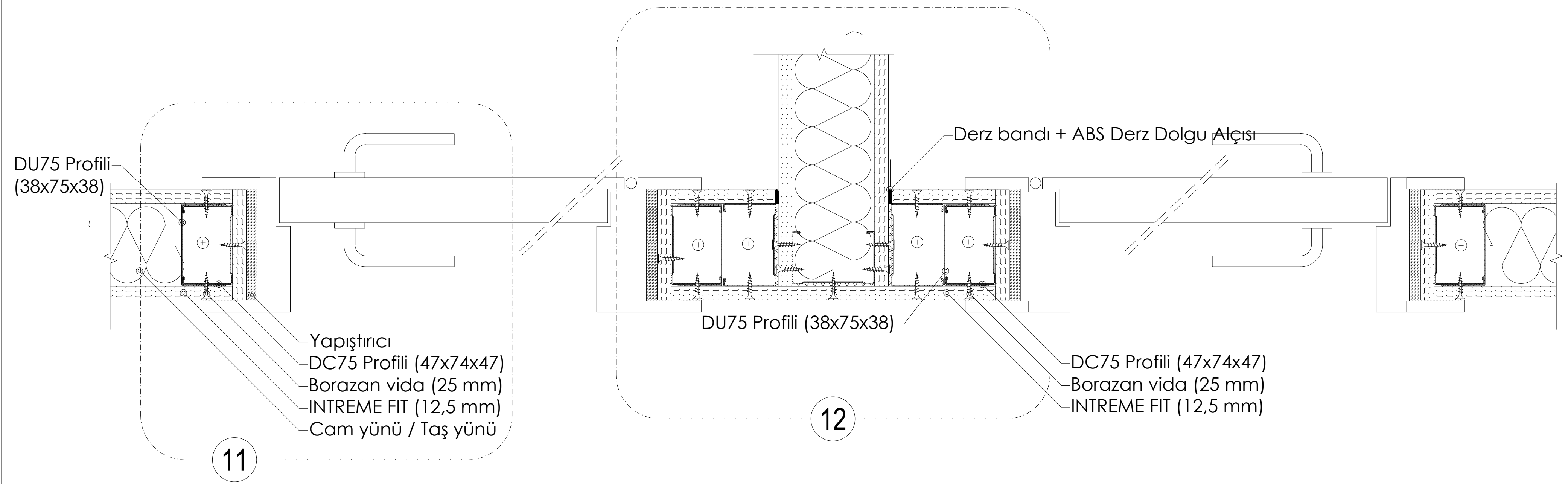
PLAN: TEK İSKELET SİSTEMİ KAPI DETAYI (YAPIŞTIRMA)
