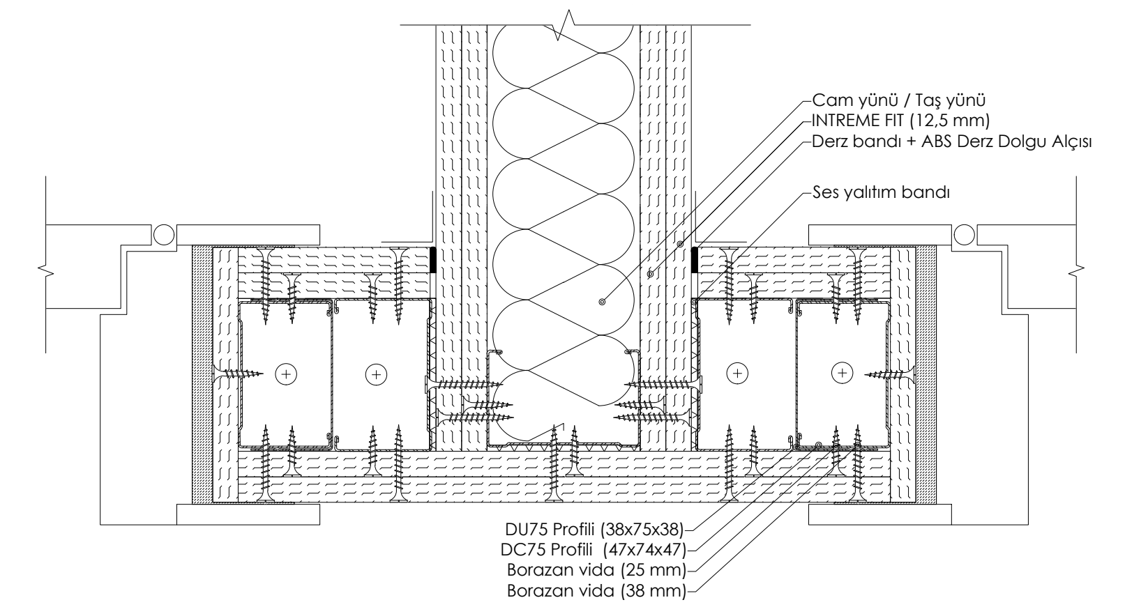
DETAY 12: TEK İSKELET SİSTEMİ KAPI PLANI (YAPIŐTIRMA)
