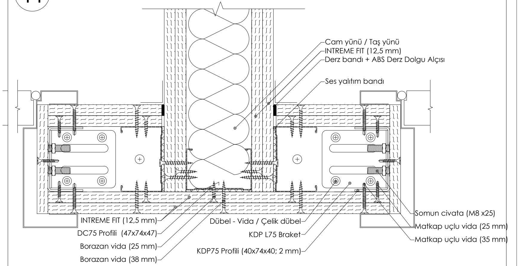
DETAY 14: TEK İSKELET SİSTEMİ KAPI DESTEK PROFİLİ DETAYI
