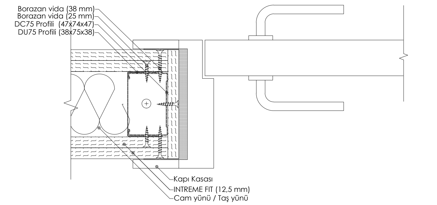
DETAY 11: TEK İSKELET SİSTEMİ KAPI PLANI (YAPIŐTIRMA)
