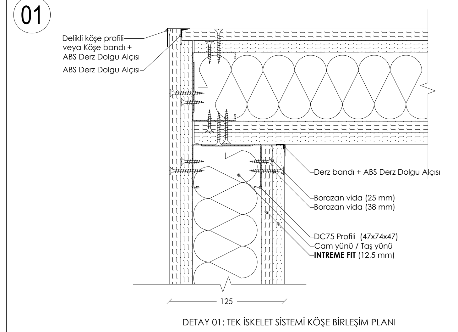
DETAY 01: TEK İSKELET SİSTEMİ KÖŞE BİRLEŞİM PLANI
