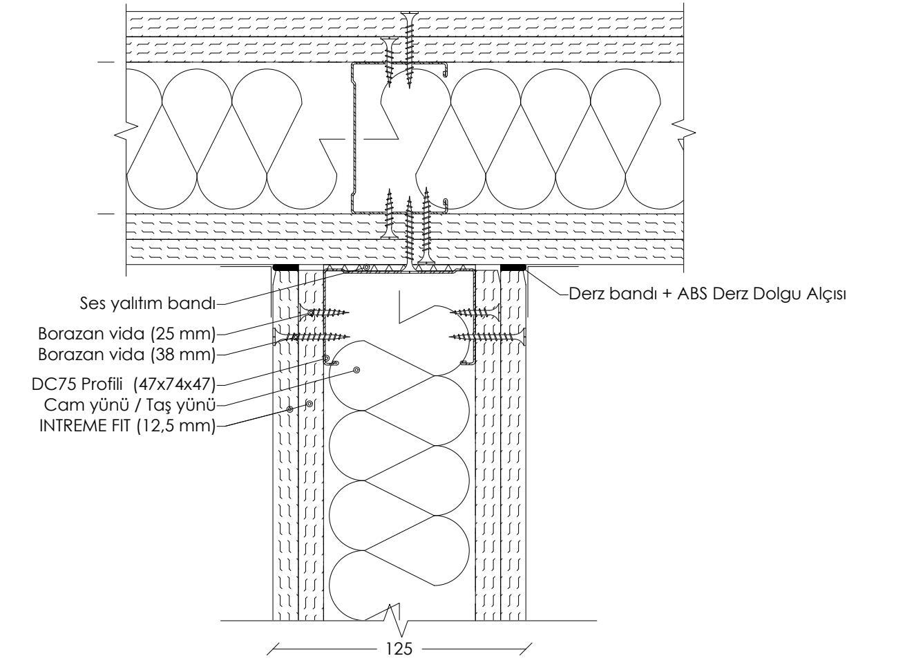
DETAY 05: TEK İSKELET SİSTEMİ BİRLEŞİM PLANI
