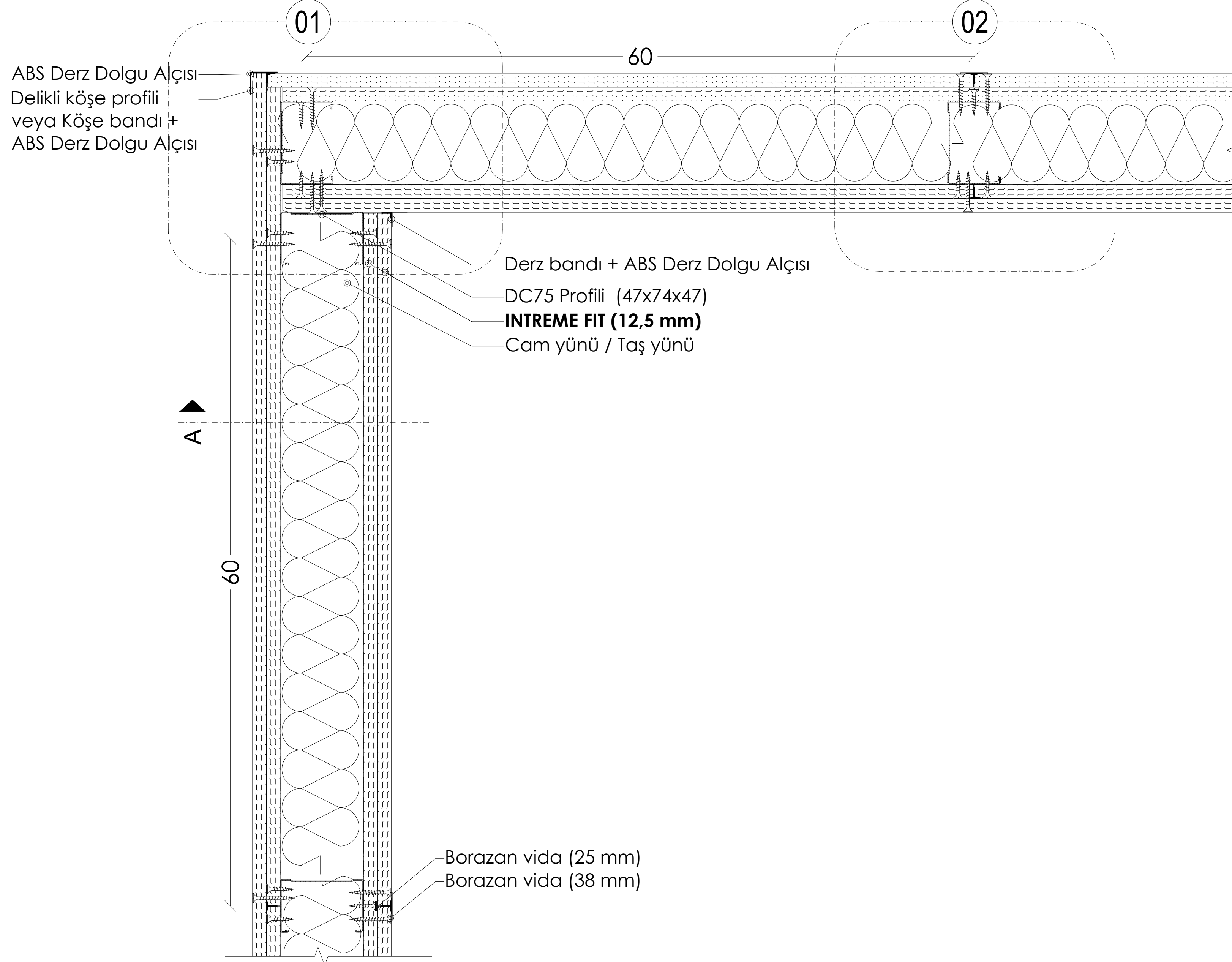
PLAN: TEK İSKELET SİSTEMİ KÖŞE BİRLEŞİMİ
