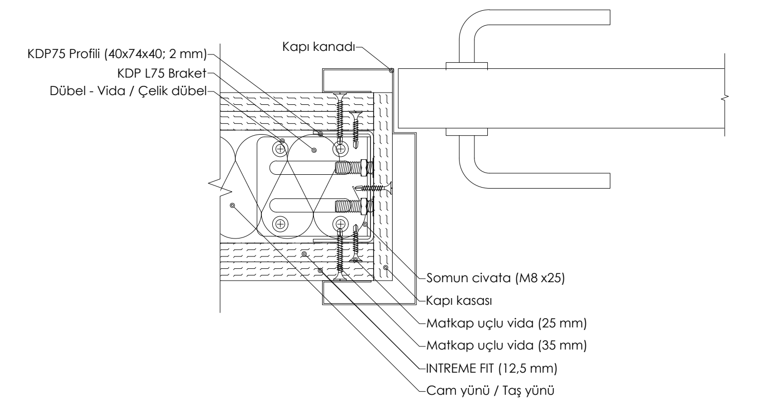
DETAY 13: TEK İSKELET SİSTEMİ KAPI DESTEK PROFİLİ DETAYI
