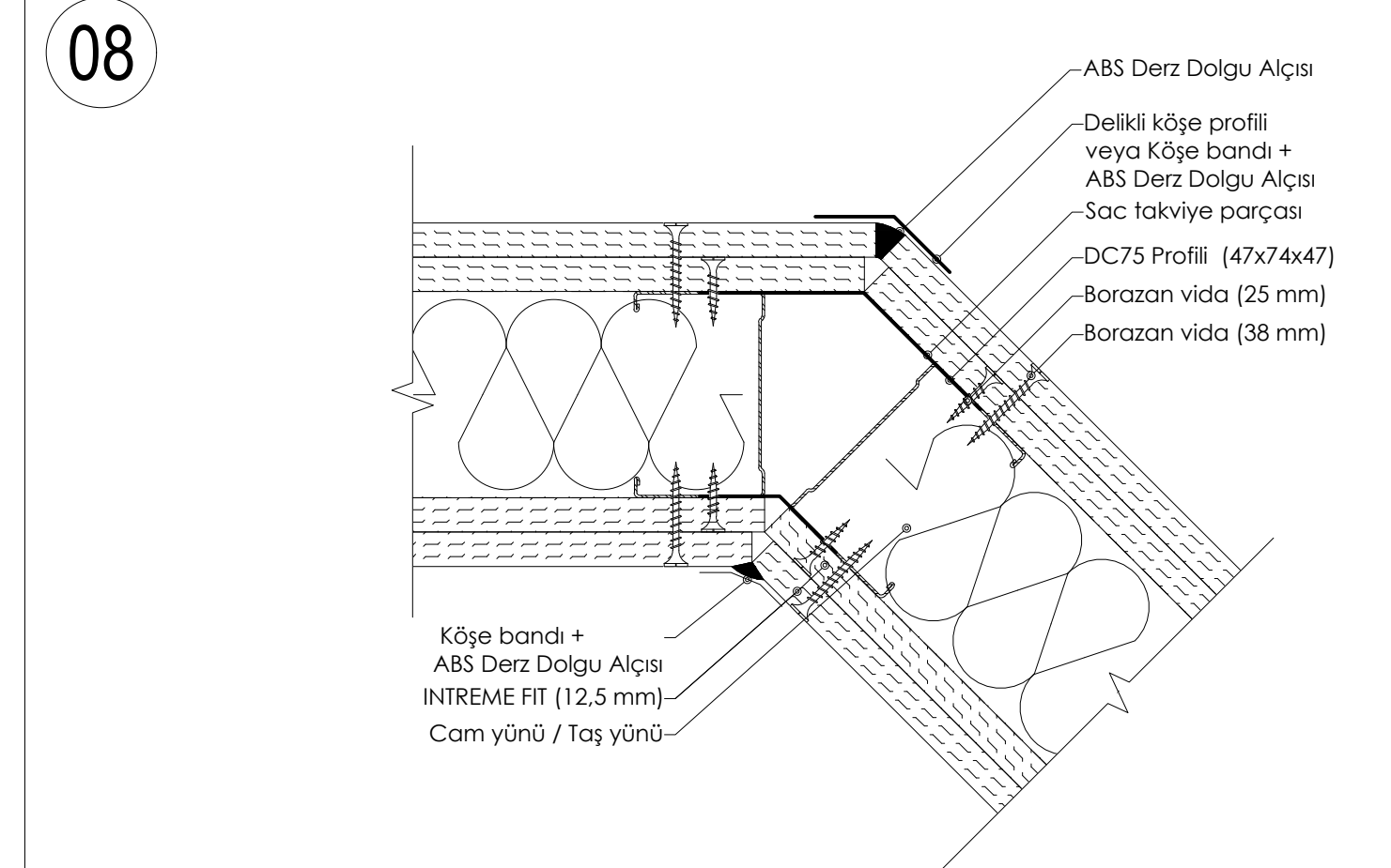
DETAY 08: TEK İSKELET SİSTEMİ 135° DUVAR BİRLEŞİMİ
