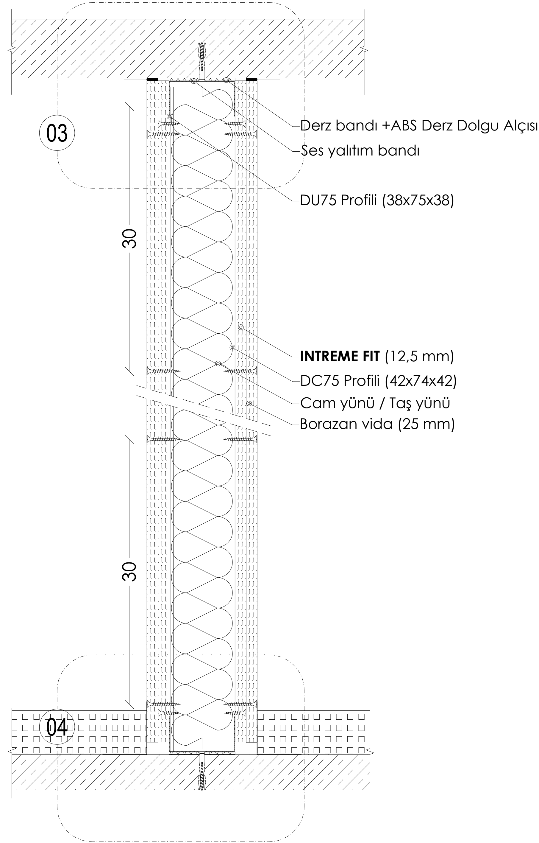
KESİT A: TEK İSKELET SİSTEMİ
