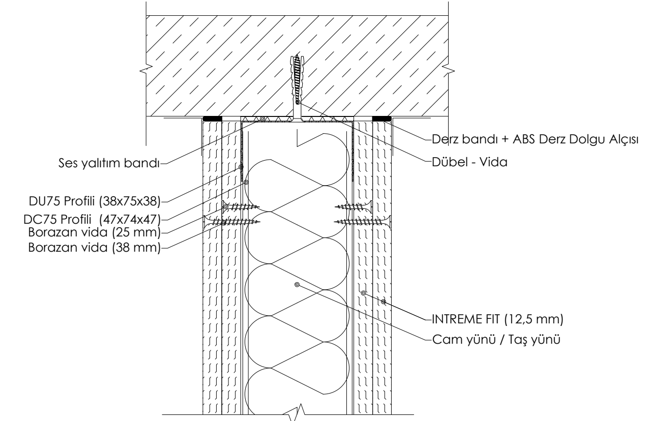
DETAY 03: TEK İSKELET SİSTEMİ TAVAN BİRLEŞİM KESİTİ
