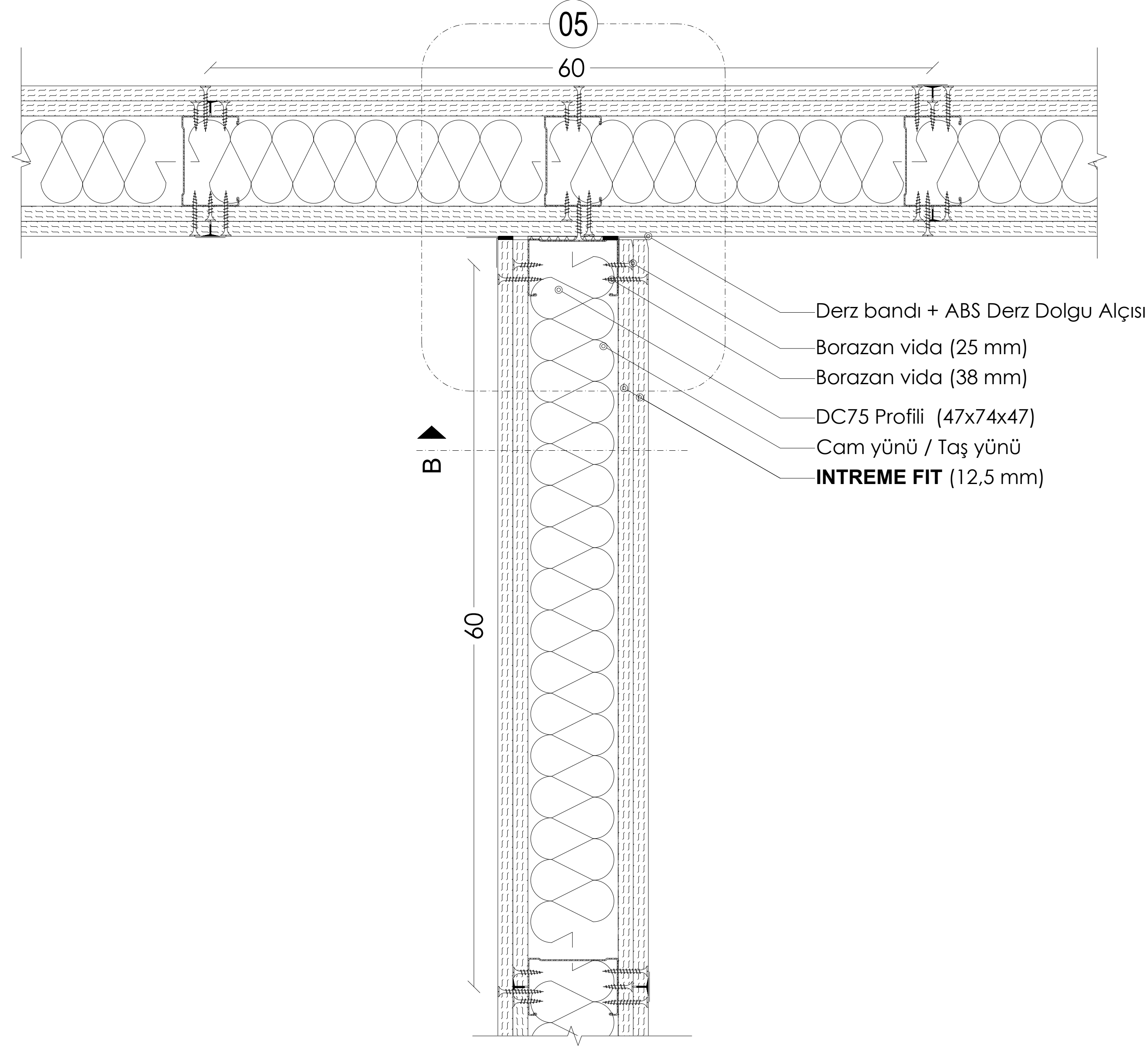
PLAN: TEK İSKELET SİSTEMİ KÖŞE BİRLEŞİMİ
