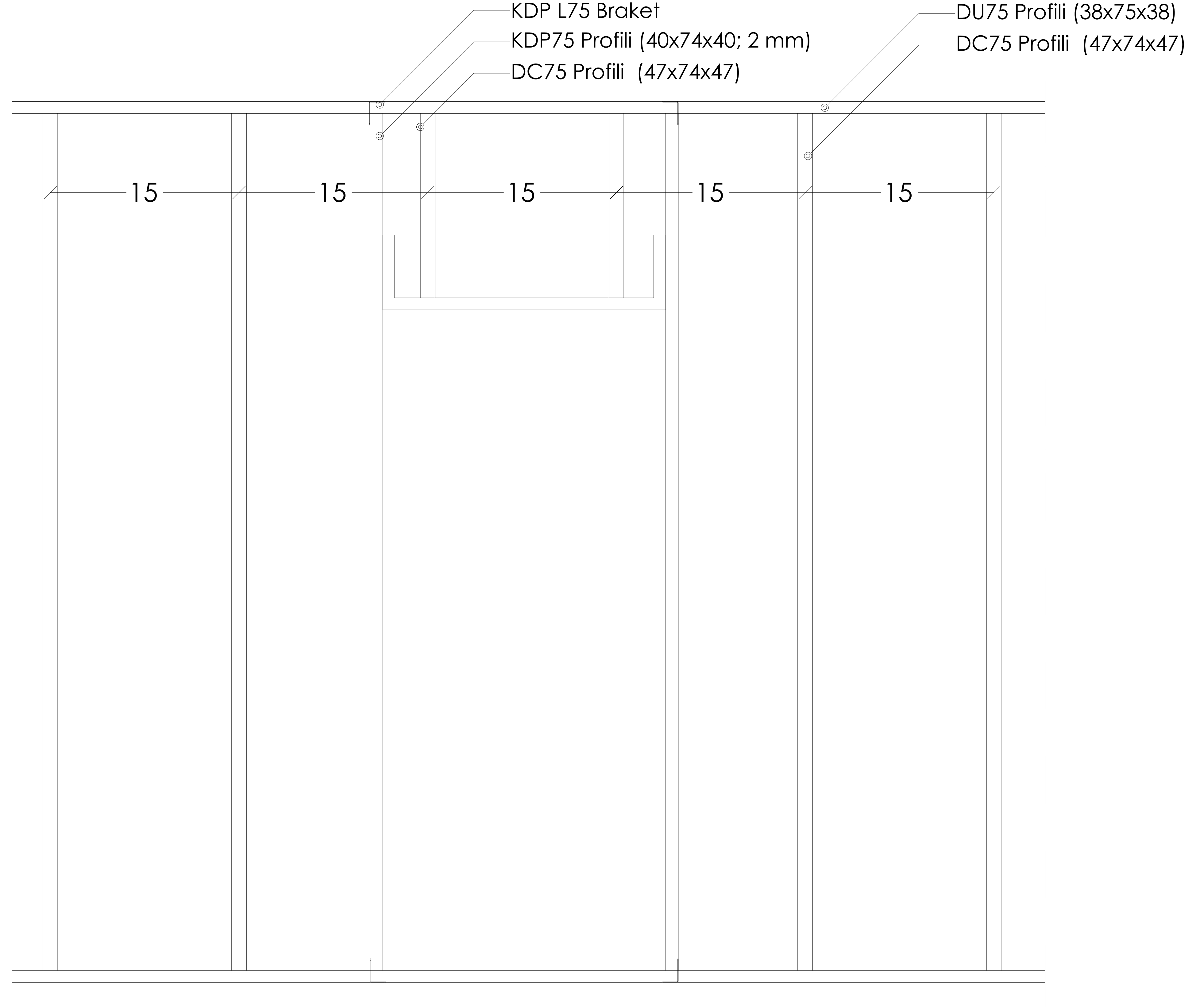
GÖRÜNÜŞ: TEK İSKELET SİSTEMİ KAPI DESTEK PROFİLİ DETAYI
