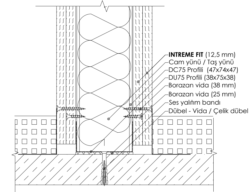
DETAY 04: TEK İSKELET SİSTEMİ ZEMİN BİRLEŞİM KESİTİ
