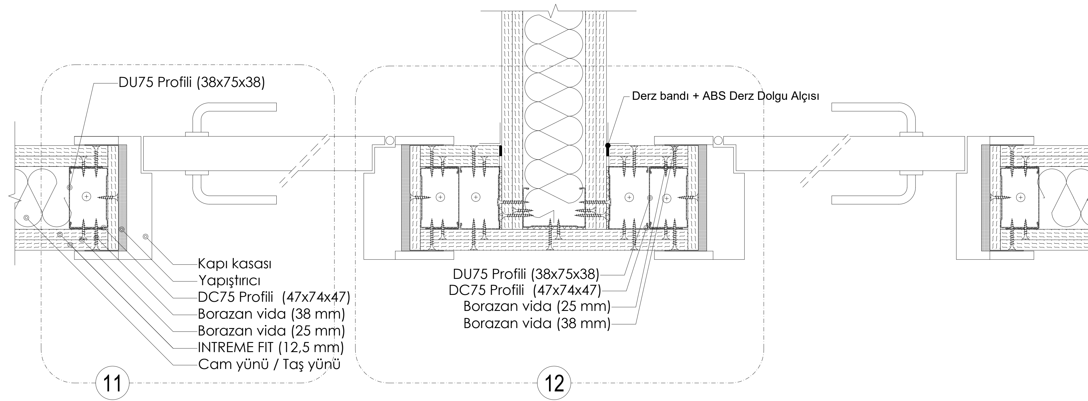
PLAN: TEK İSKELET SİSTEMİ KAPI DETAYI (YAPIŐTIRMA)
