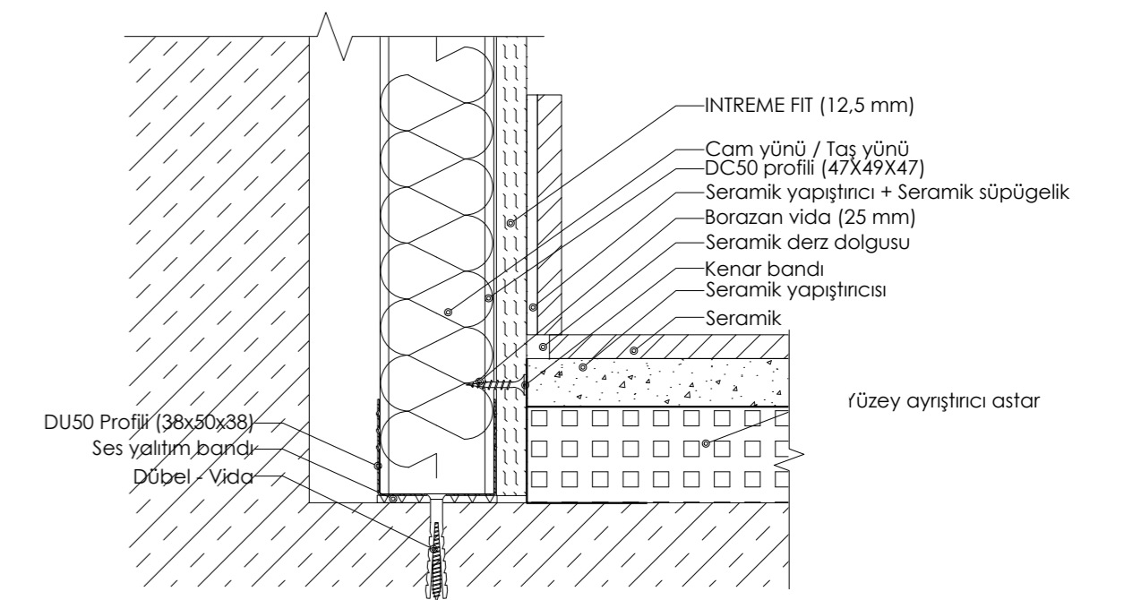
DETAY 04: METAL İSKELETLİ GİYDİRME DUVAR (BÖLME DUVAR PROFİLLERİ İLE DÖŞEME ÜZERİNE) SERAMİK DETAYI
