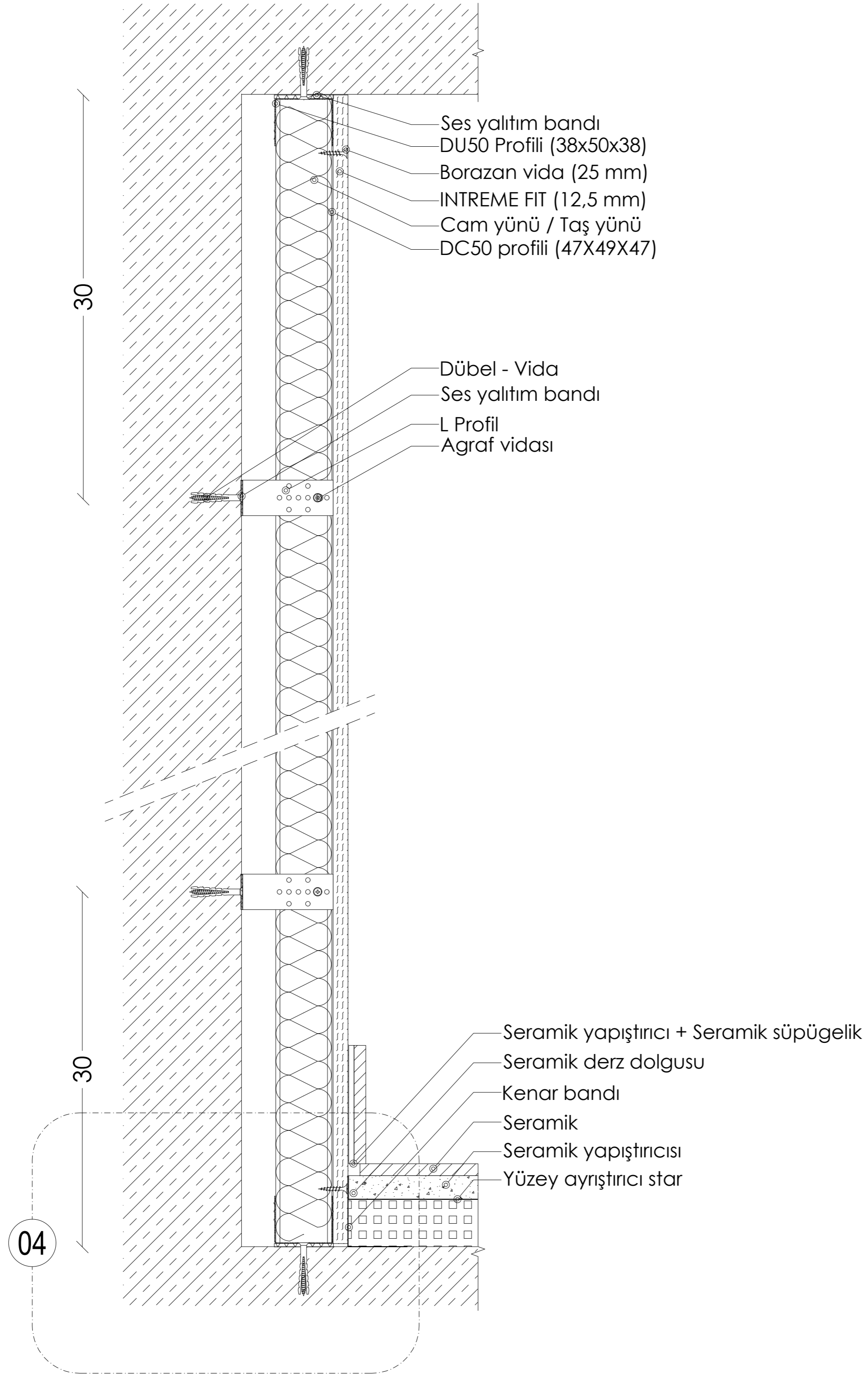
KESİT B: METAL İSKELETLİ GİYDİRME DUVAR (BÖLME DUVAR PROFİLLERİ İLE DÖŞEME ÜZERİNE) SERAMİK DETAYI
