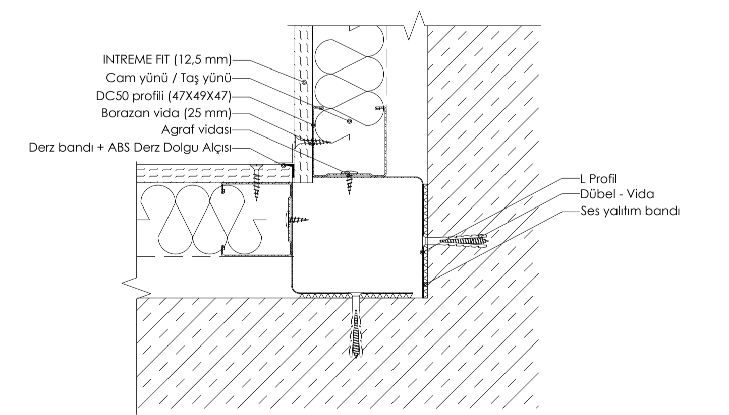
DETAY 03: METAL İSKELETLİ GİYDİRME DUVAR (BÖLME DUVAR PROFİLLERİ İLE) İÇ KÖŞE BİRLEŞİM PLANI
