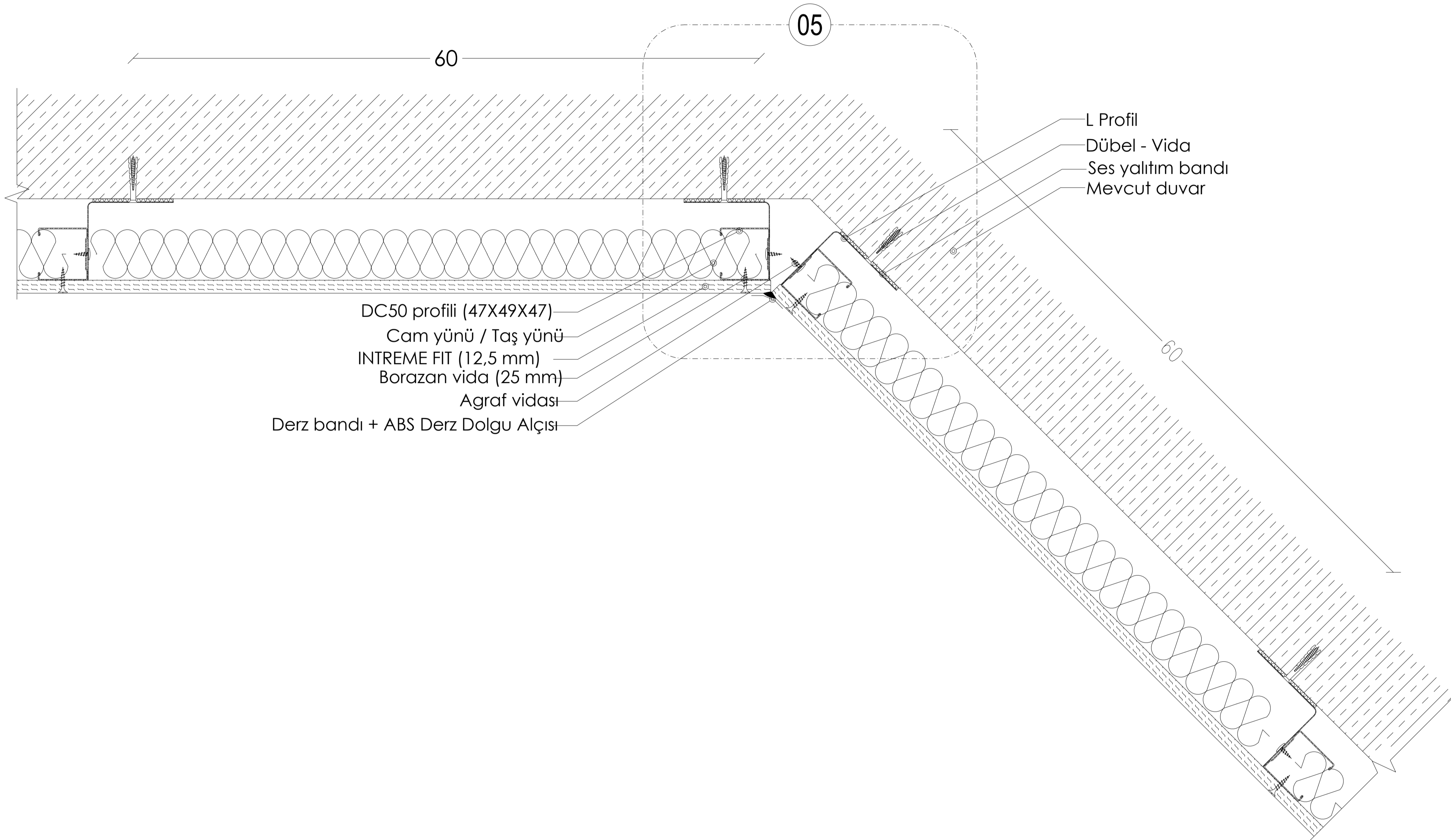
PLAN:PLAN: METAL İSKELETLİ GİYDİRME DUVAR (BÖLME DUVAR PROFİLLERİ İLE) 135° BİRLEŞİMİ
