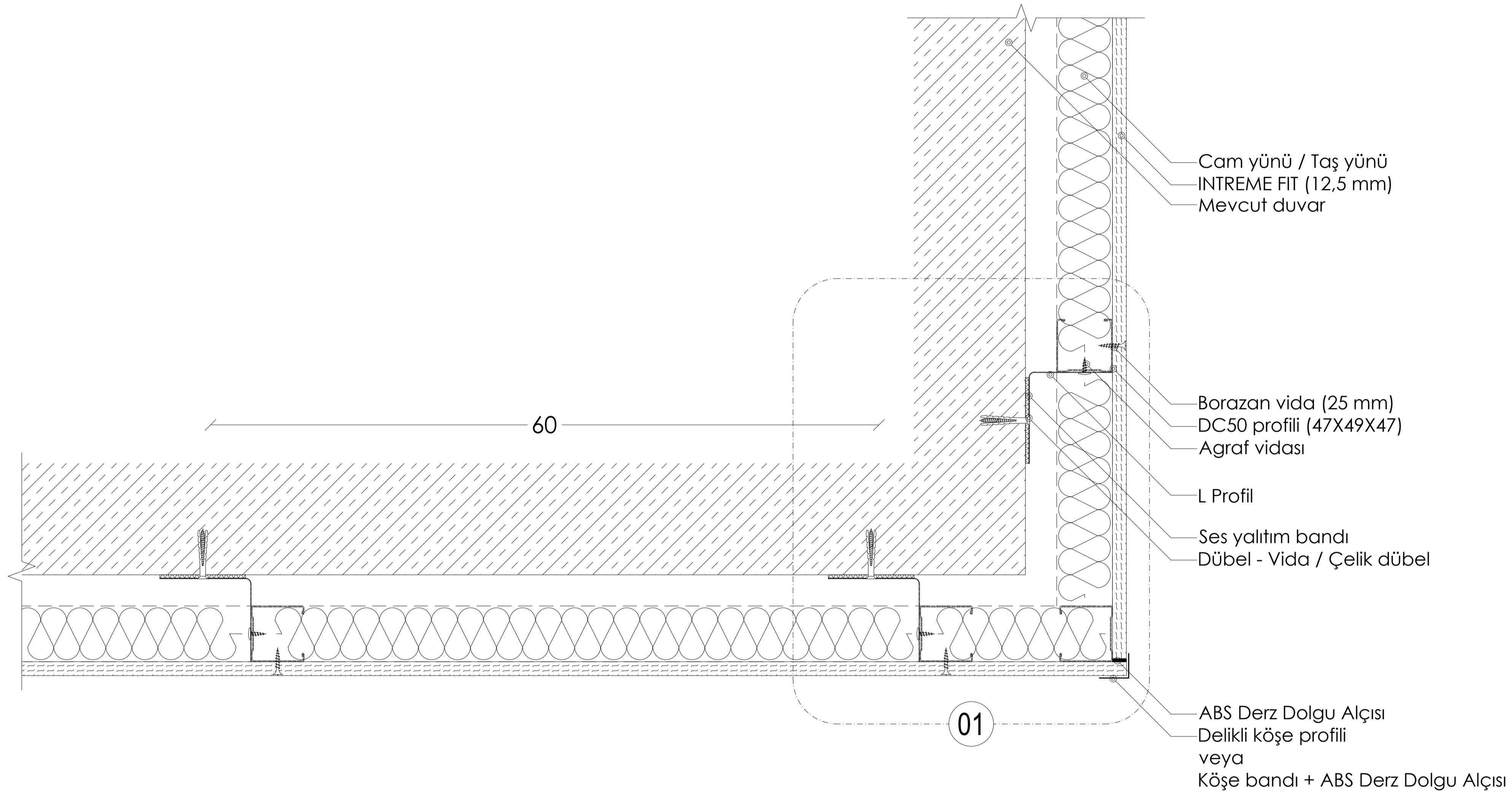
PLAN: METAL İSKELETLİ GİYDİRME DUVAR ( BÖLME DUVAR PROFİLLERİ İLE ) DIŞ KÖŞE BİRLEŞİMİ
