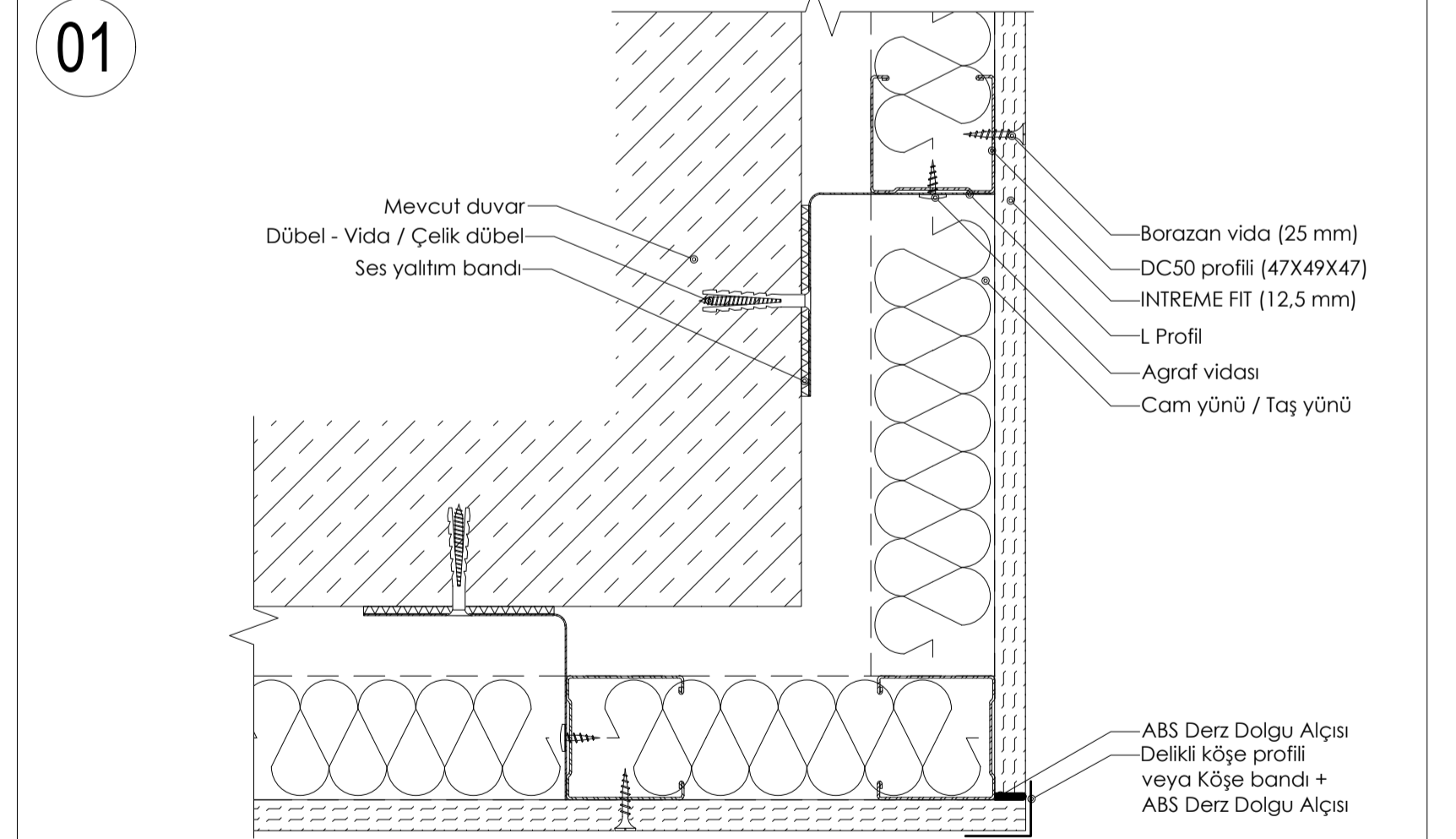
DETAY 01: METAL İSKELETLİ GİYDİRME DUVAR (BÖLME DUVAR PROFİLLERİ İLE) DIŞ KÖŞE BİRLEŞİM PLANI
