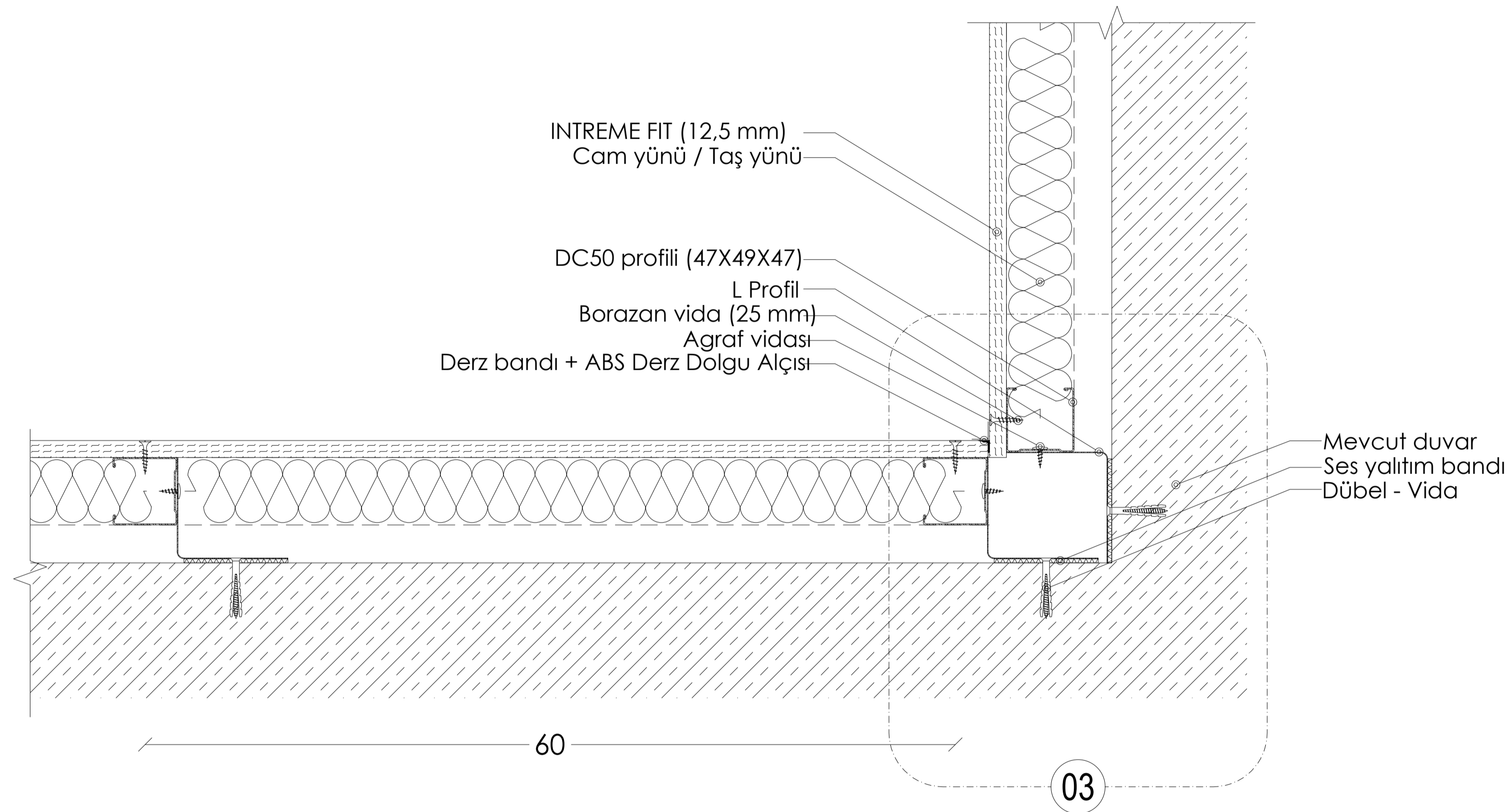
PLAN:PLAN: METAL İSKELETLİ GİYDİRME DUVAR (BÖLME DUVAR PROFİLLERİ İLE) İÇ KÖŞE BİRLEŞİMİ
