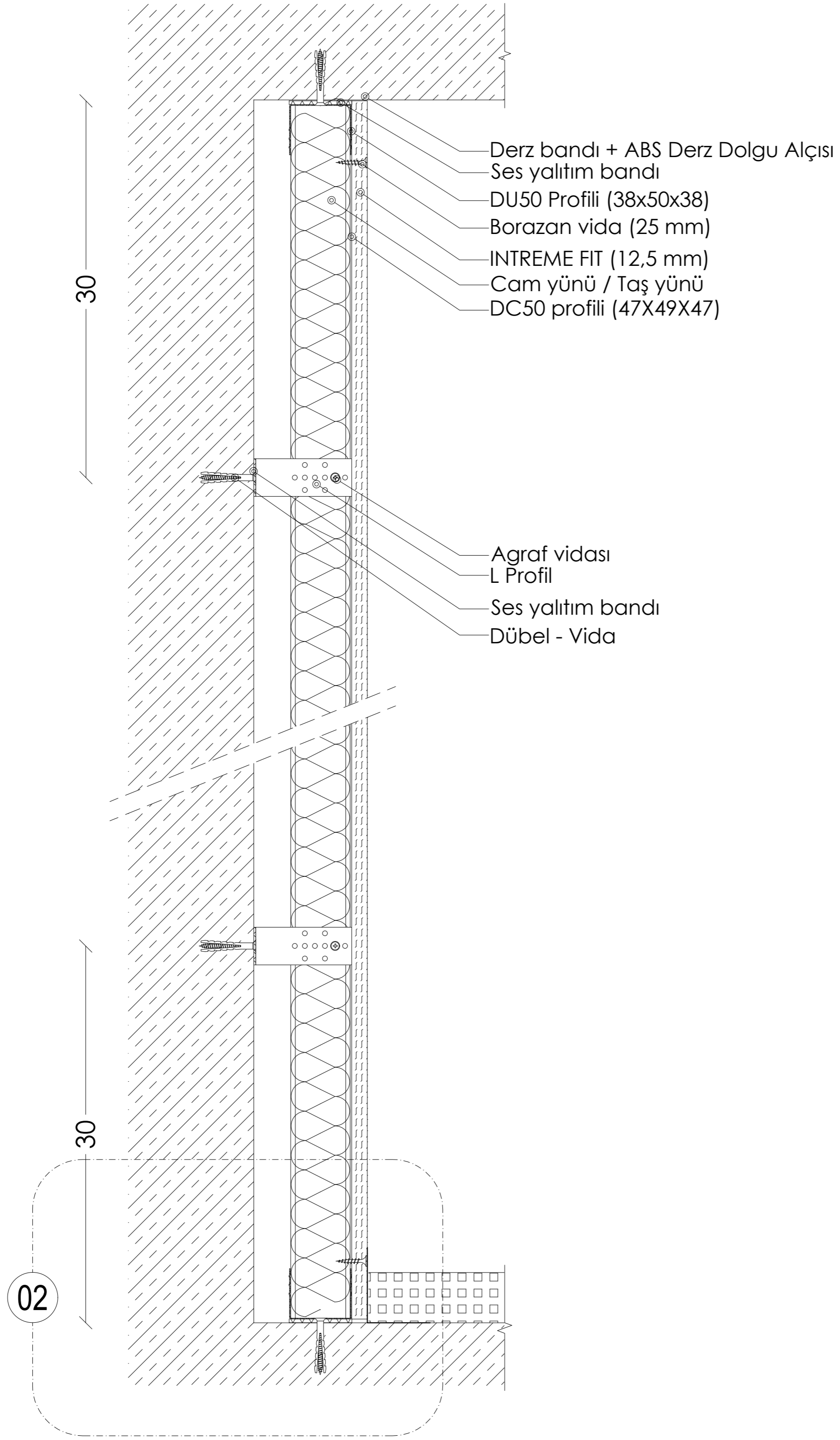
KESİT A: METAL İSKELETLİ GİYİRME DUVAR (BÖLME DUVAR PROFİLLERİ İLE DÖŞEME ÜZERİNE)
