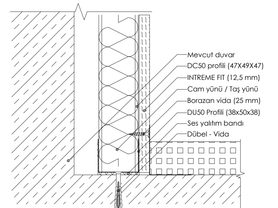
DETAY 02: METAL İSKELETLİ GİYİRME DUVAR (BÖLME DUVAR PROFİLLERİ İLE) DÖŞEME ÜZERİNE ZEMİN BİRLEŞİM KESİTİ
