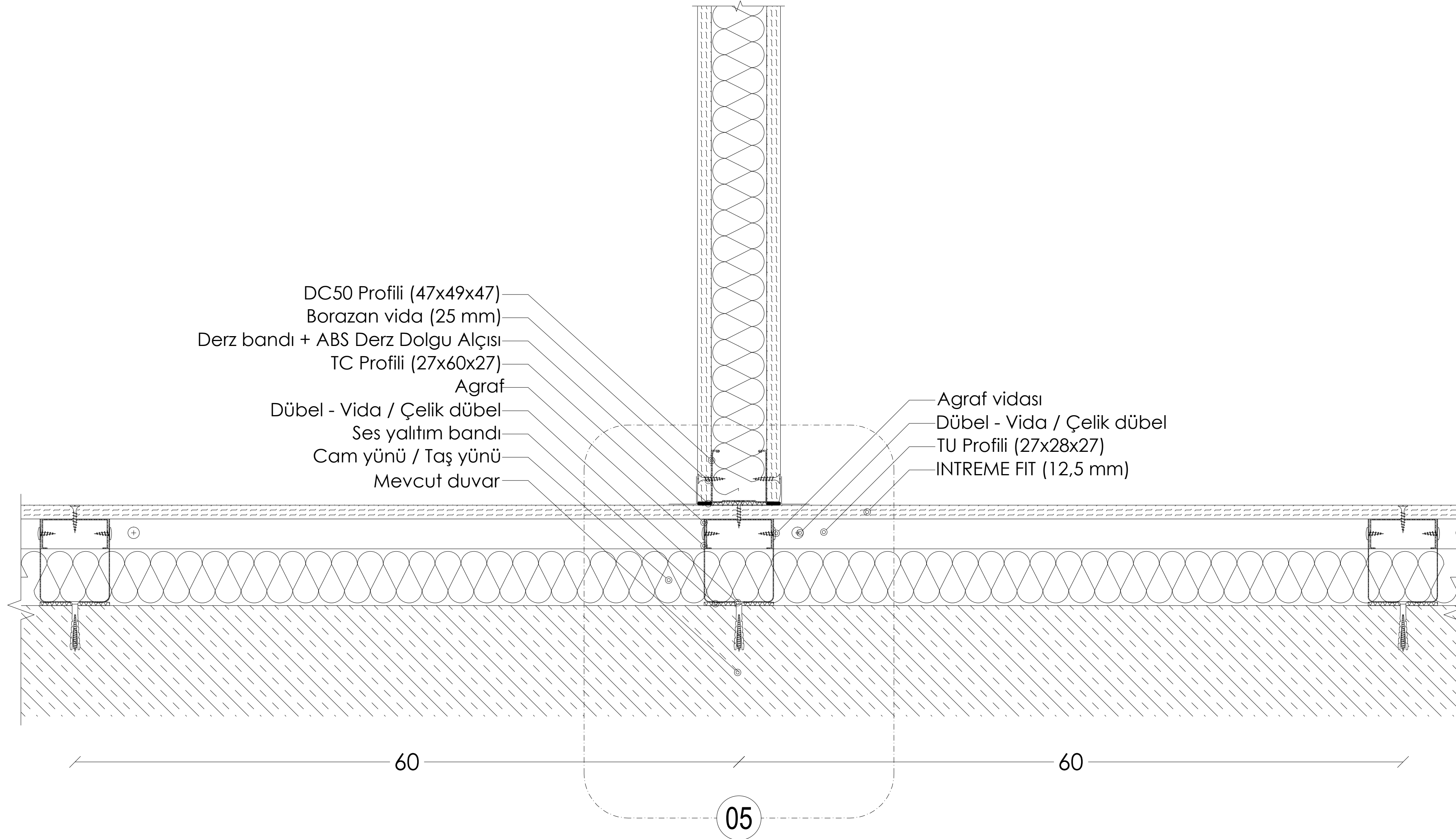
PLAN: METAL İSKELETLİ (TAVAN PROFİLLERİ İLE) GİYDİRME DUVAR - BÖLME DUVAR BİRLEŞİMİ
