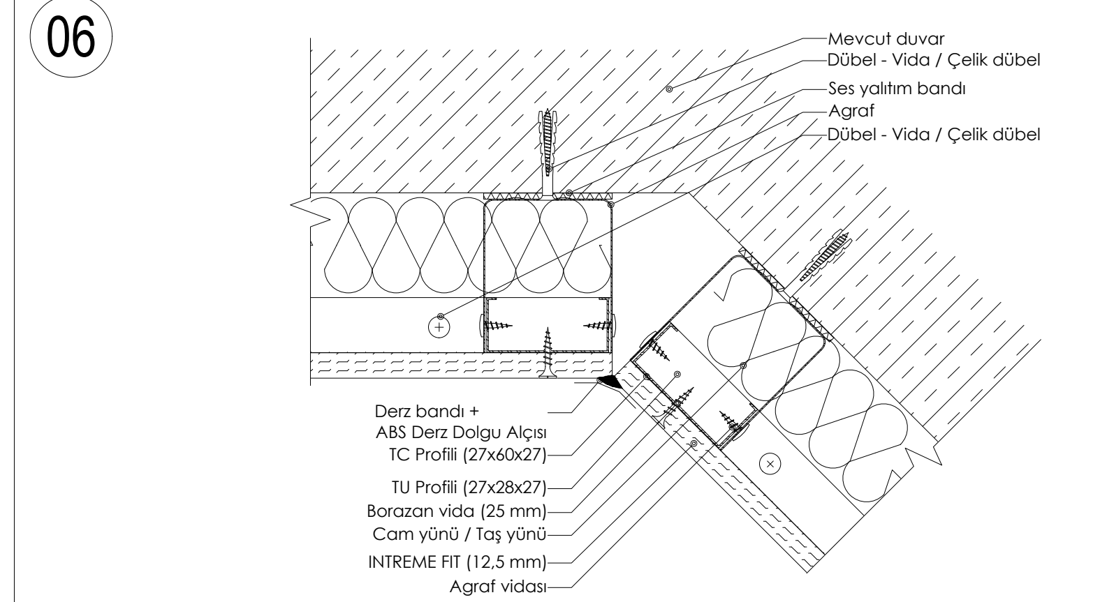
DETAY 06: METAL İSKELETLİ (TAVAN PROFİLLERİ İLE) GİYDİRME DUVAR - BÖLME DUVAR BİRLEŞİM PLANI
