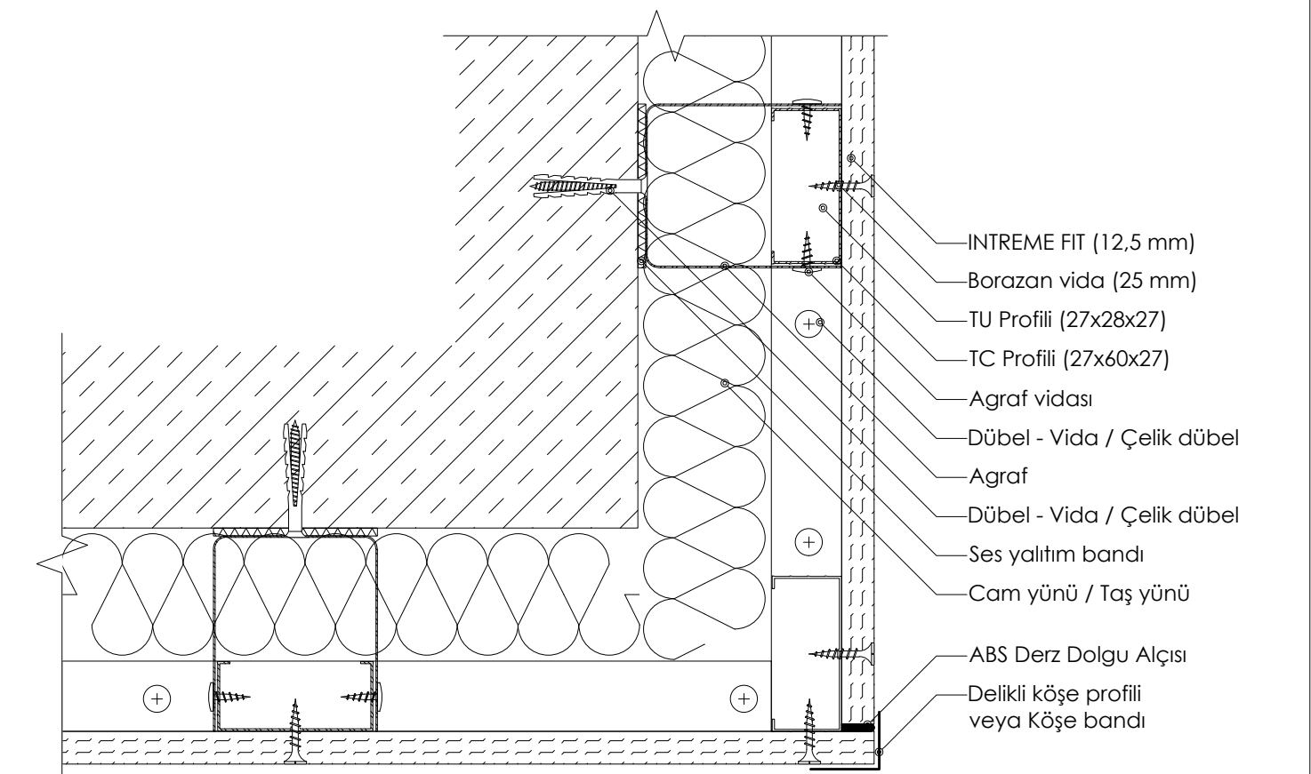
DETAY 01: METAL İSKELETLİ GİYDİRME DUVAR (TAVAN PROFİLLERİ İLE) DIŞ KÖŞE BİRLEŞİM PLANI
