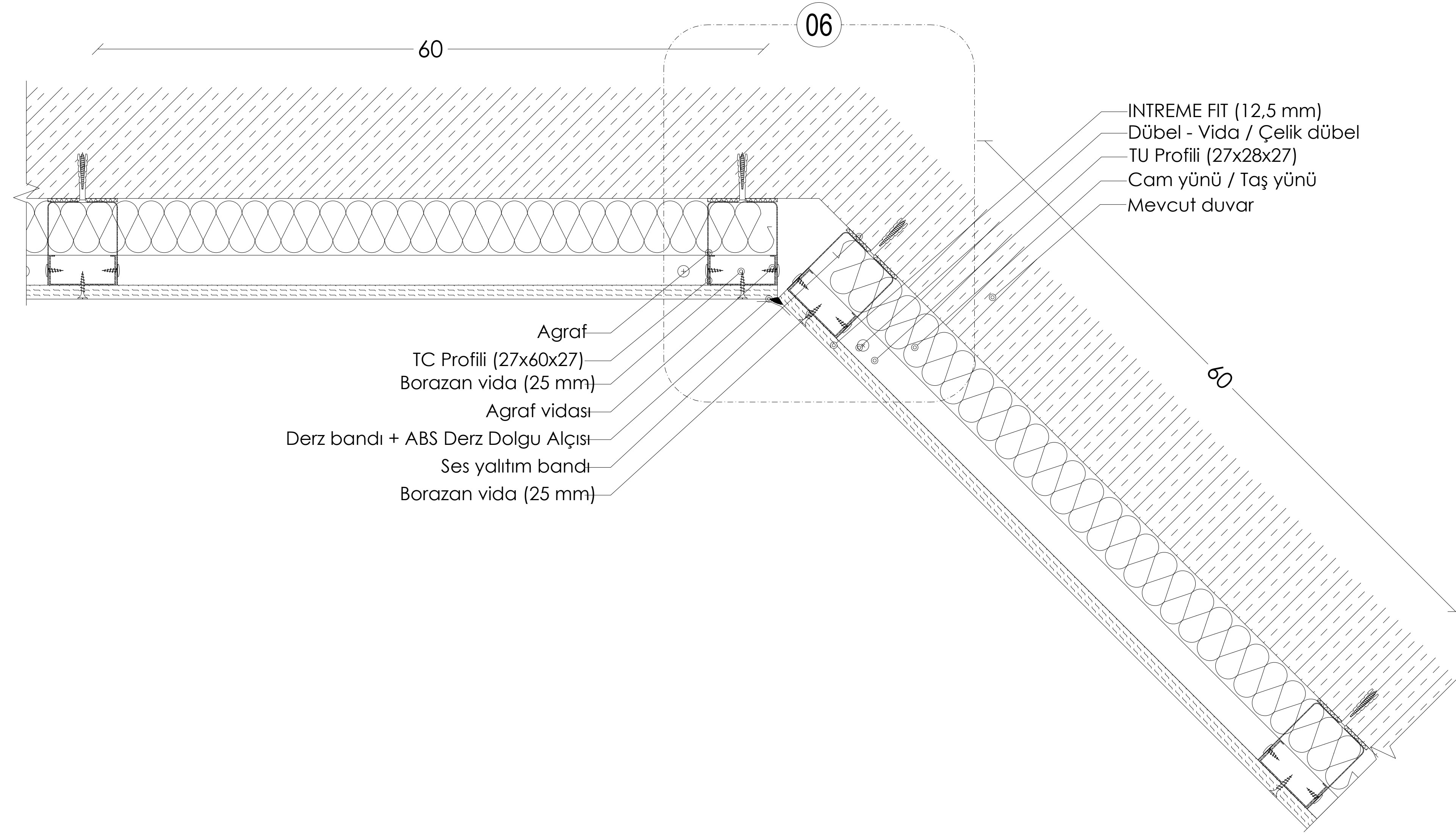
PLAN: METAL İSKELETLİ GİYDİRME DUVAR (TAVAN PROFİLLERİ İLE) 135° BİRLEŞİMİ
