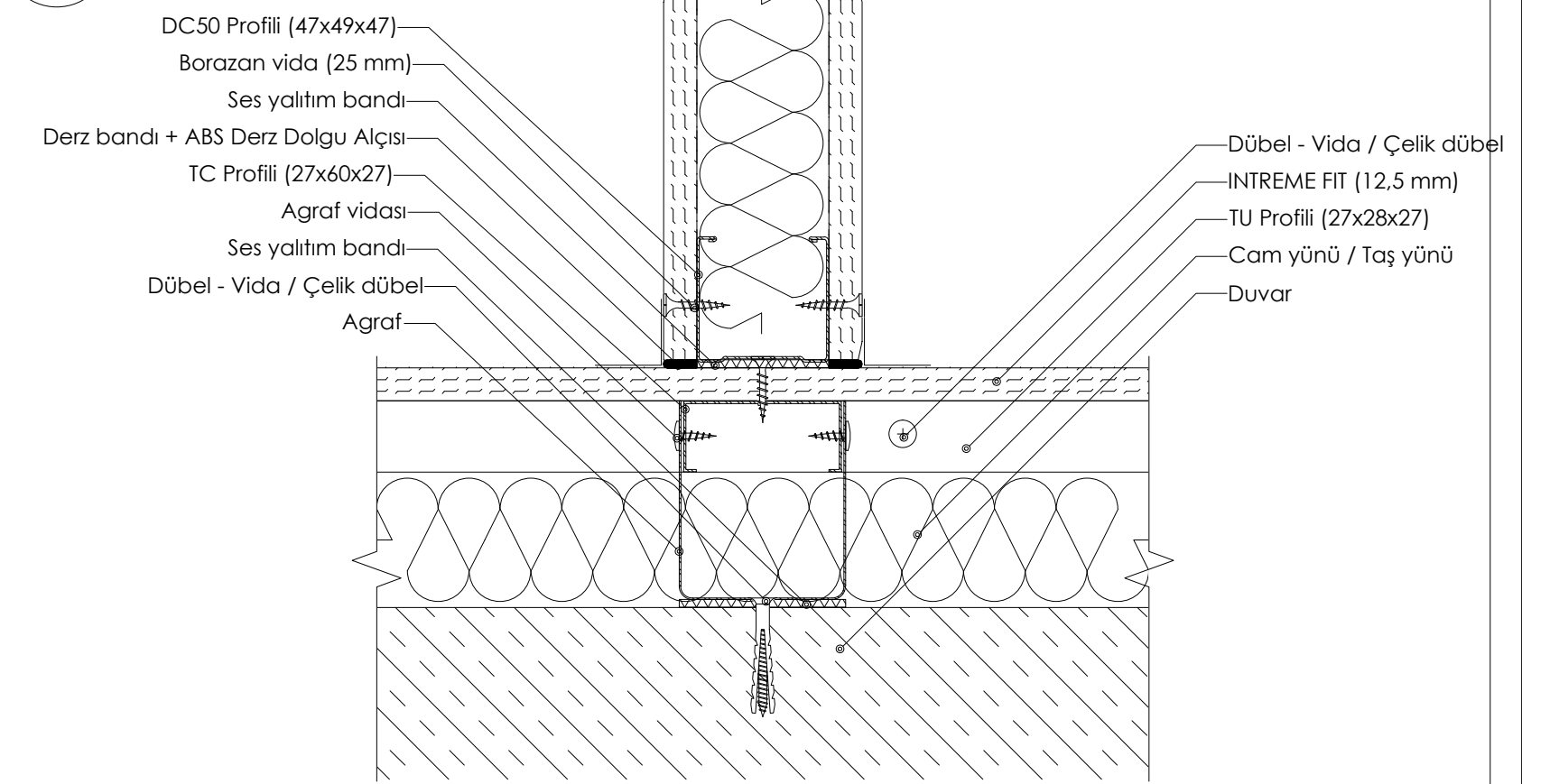
DETAY 05: METAL İSKELETLİ (TAVAN PROFİLLERİ İLE) GİYDİRME DUVAR - BÖLME DUVAR BİRLEŞİM PLANI
