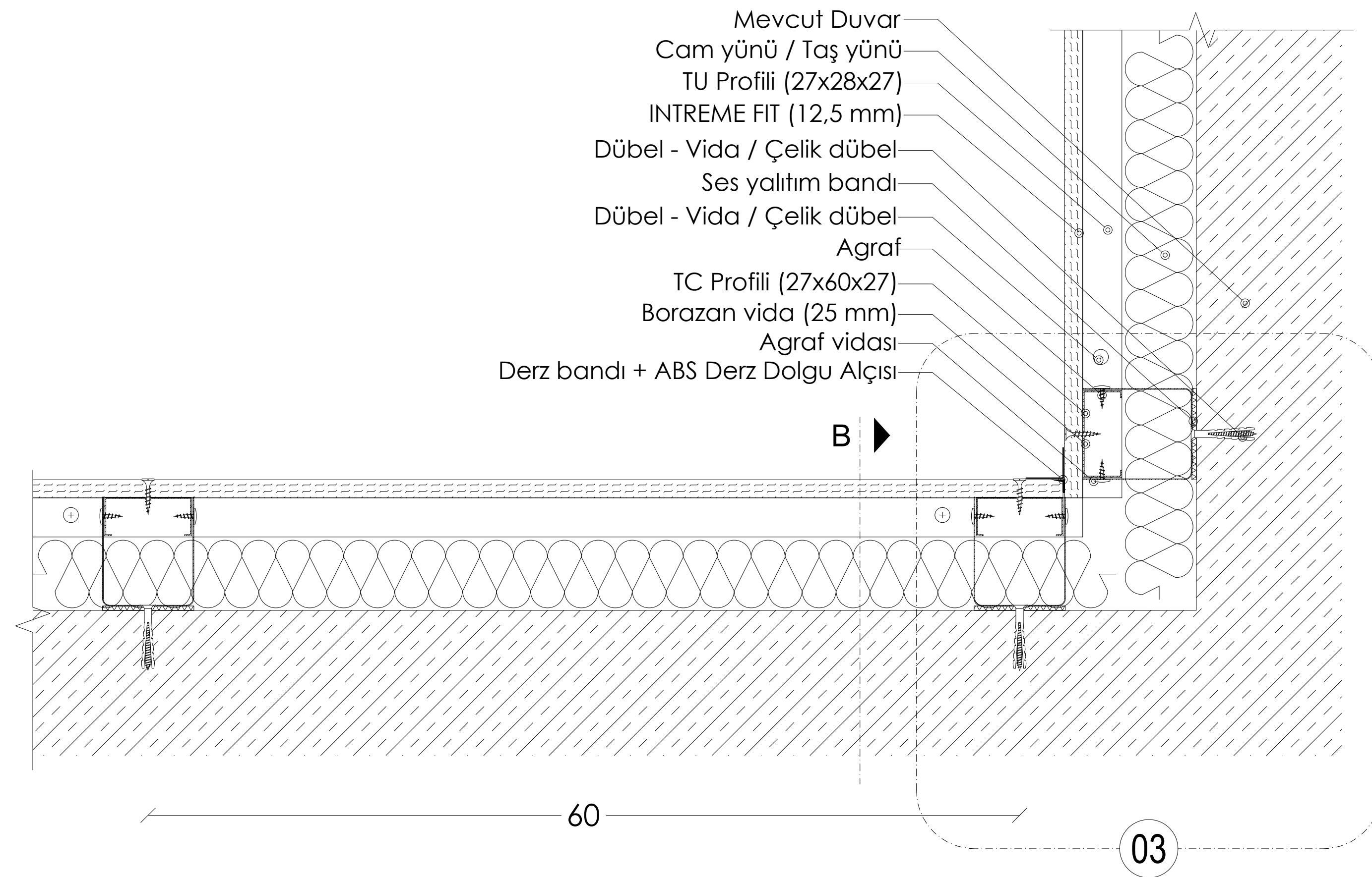
PLAN: METAL İSKELETLİ GİYDİRME DUVAR (TAVAN PROFİLLERİ İLE) İÇ KÖŞE BİRLEŞİMİ
