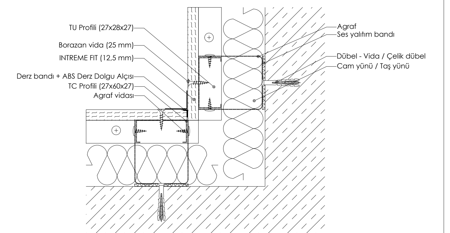
DETAY 03: METAL İSKELETLİ GİYDİRME DUVAR (TAVAN PROFİLLERİ İLE) İÇ KÖŞE BİRLEŞİM PLANI
