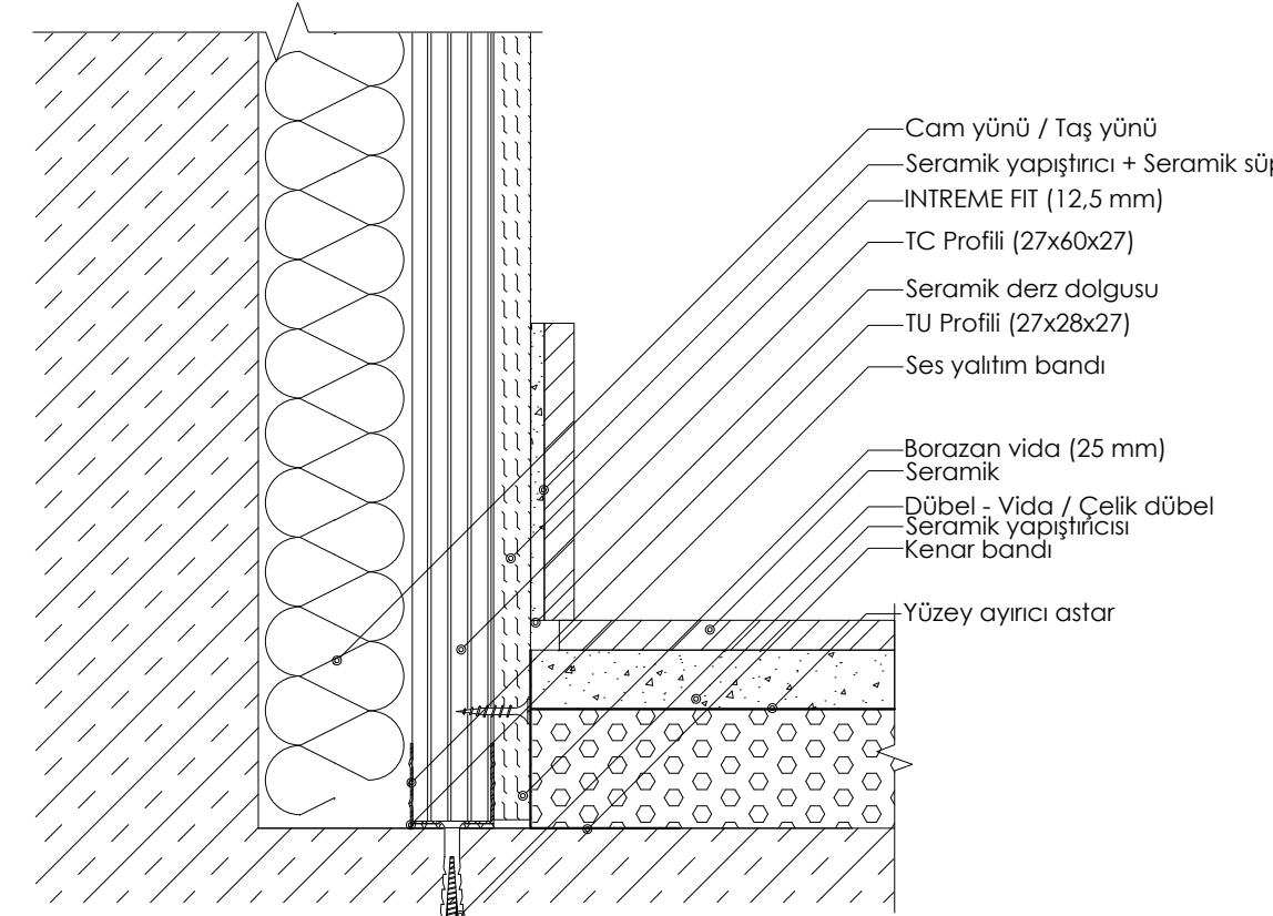
DETAY 04: METAL İSKELETLİ GİYDİRME DUVAR (TAVAN PROFİLLERİ İLE DÖŞEME ÜZERİNE) SERAMİK KAPLAMA
