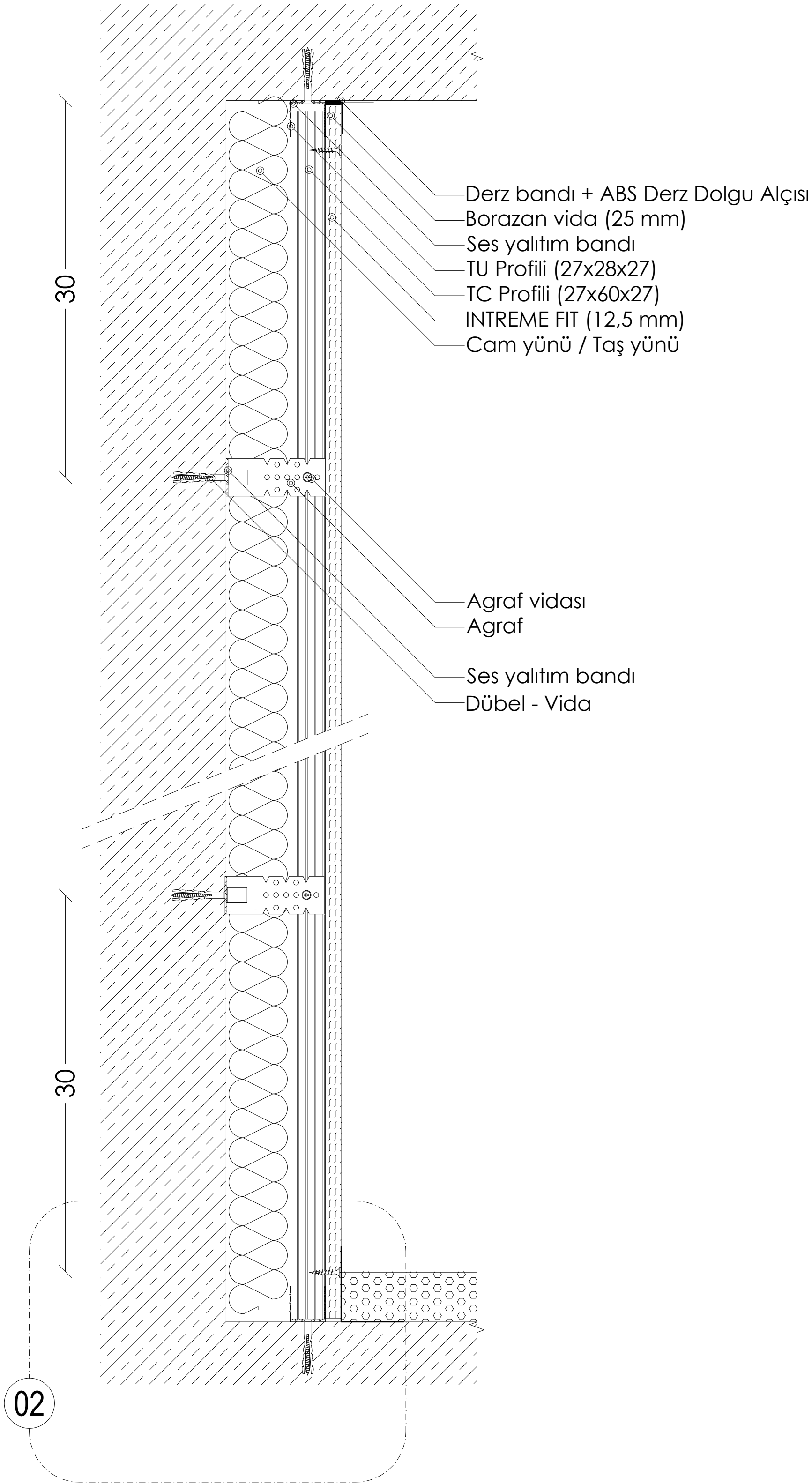
KESİT A: METAL İSKELETLİ GİYDİRME DUVAR (TAVAN PROFİLLERİ İLE DÖŞEME ÜZERİNE)
