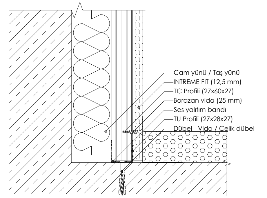
DETAY 02: METAL İSKELETLİ GİYDİRME DUVAR (TAVAN PROFİLLERİ İLE DÖŞEME ÜZERİNE) ZEMİN BİRLEŞİM KESİTİ
