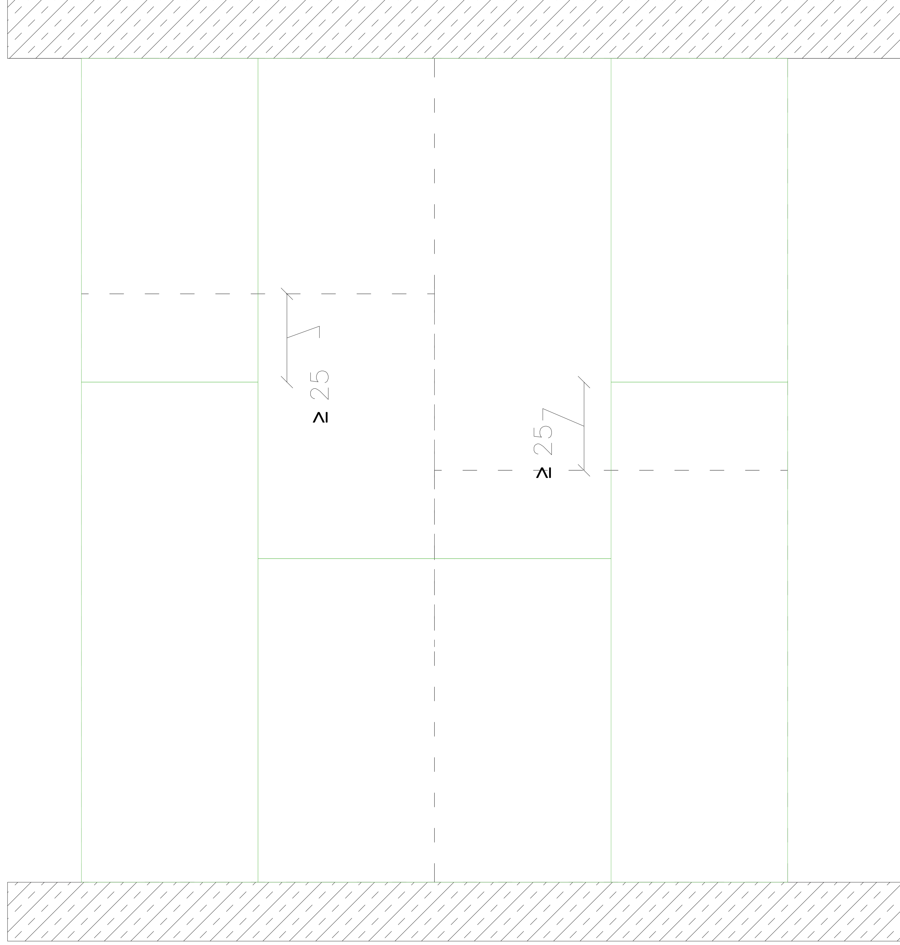
GÖRÜNÜŞ: İKİNCİ KAT INTREME FIT YERLEŞİMİ
