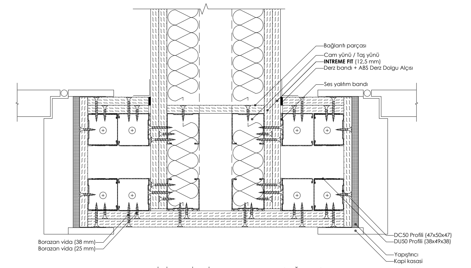
DETAY 12: ÇİFT İSKELET SİSTEMİ YAPIŞTIRMA KAPI PLANI (BAĞLANTILI)
