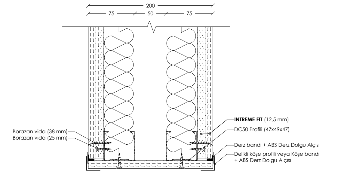
DETAY 07: ÇİFT İSKELET SİSTEMİ DİŞ DUVAR PLANI (BAĞLANTILI)
