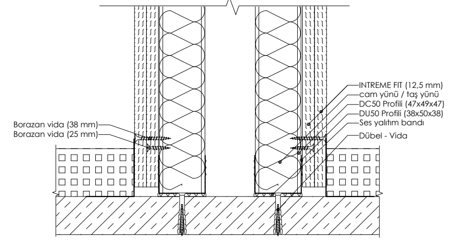
DETAY 04: ÇİFT İSKELET SİSTEMİ ZEMİN BİRLEŞİM KESİTİ (BAĞLANTILI)
