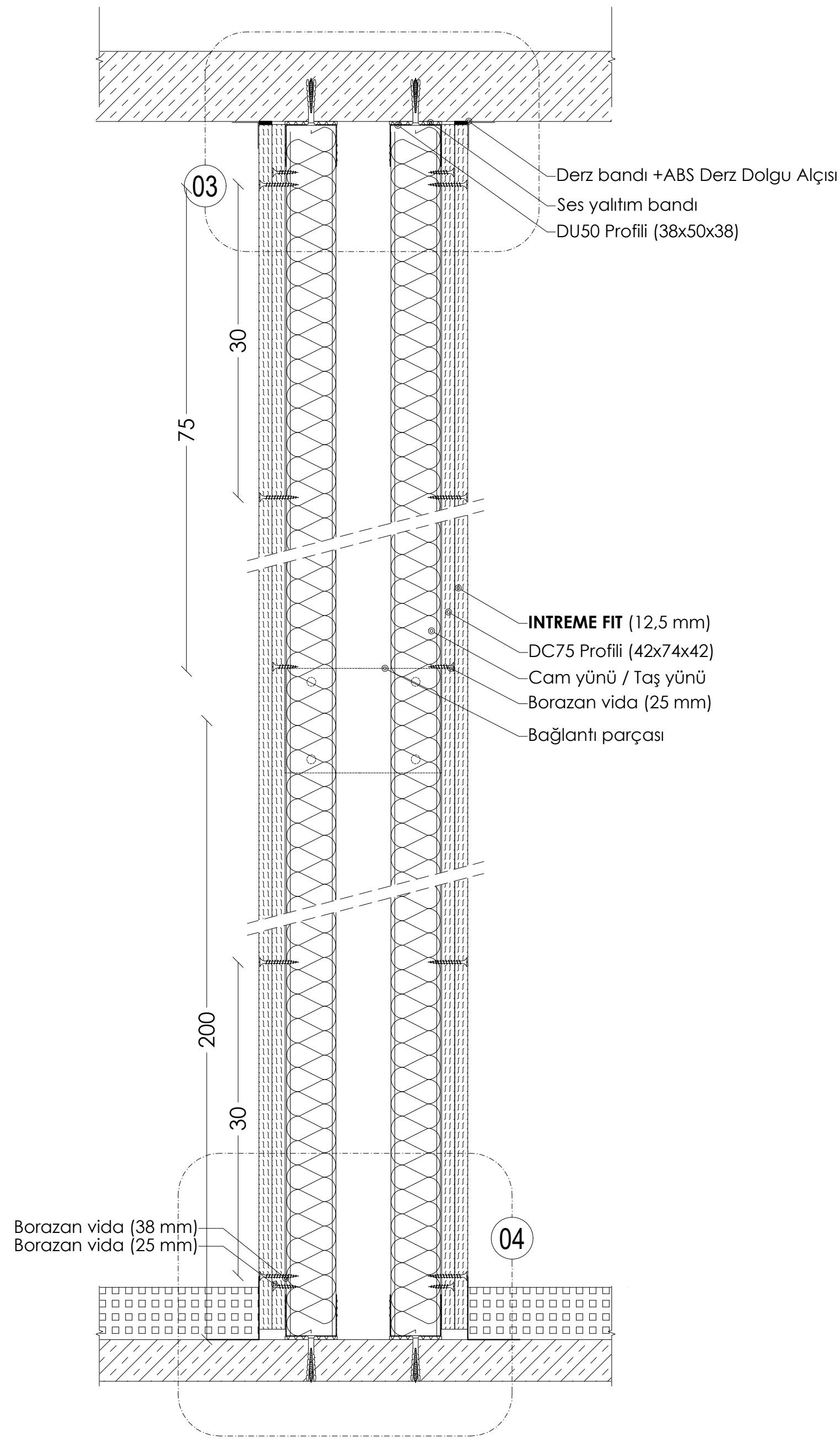
KESİT A: ÇİFT İSKELET SİSTEMİ (BAĞLANTILI)
