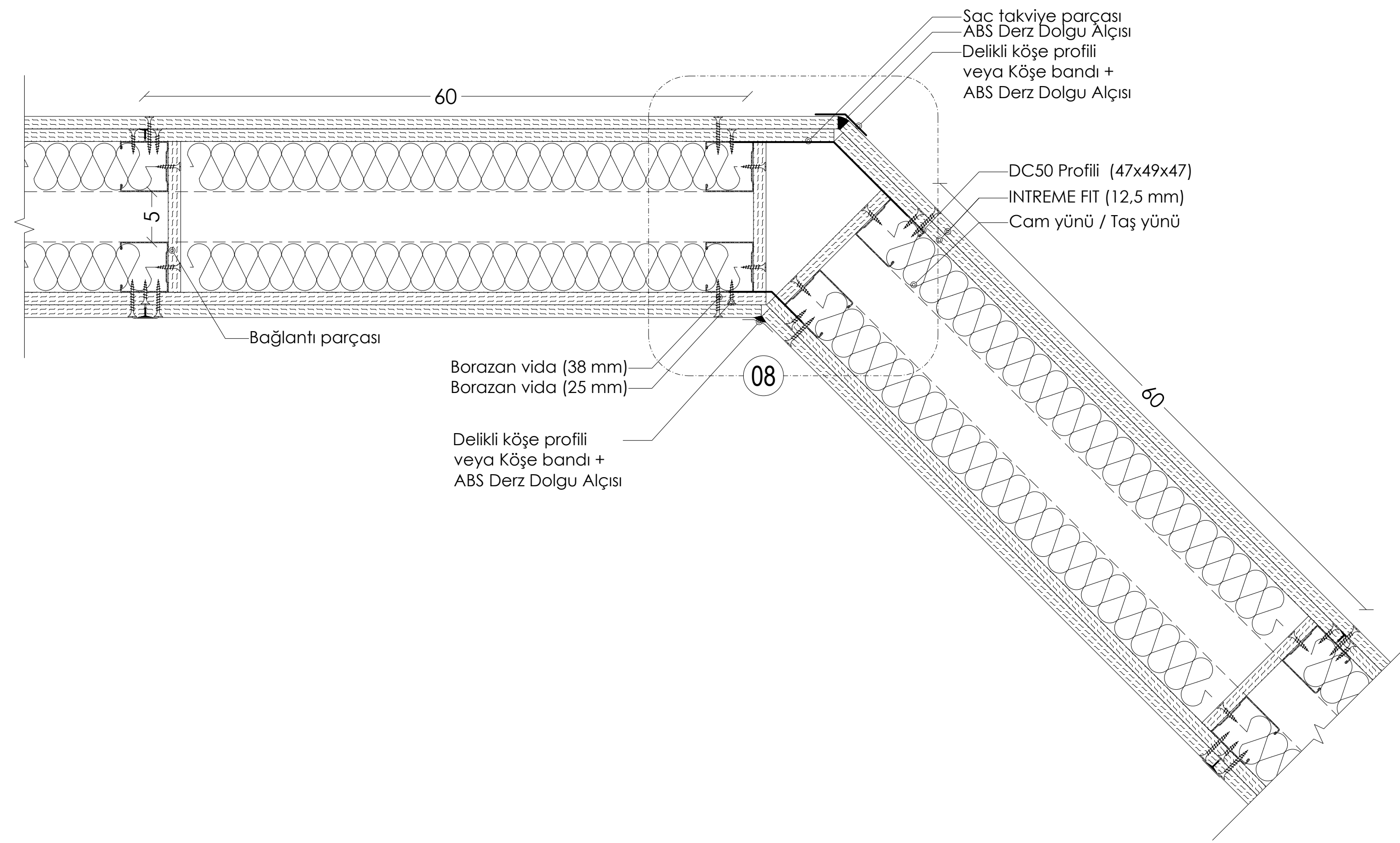
PLAN: ÇİFT İSKELET SİSTEMİ 135° DUVAR BİRLEŞİMİ (BAĞLANTILI)
