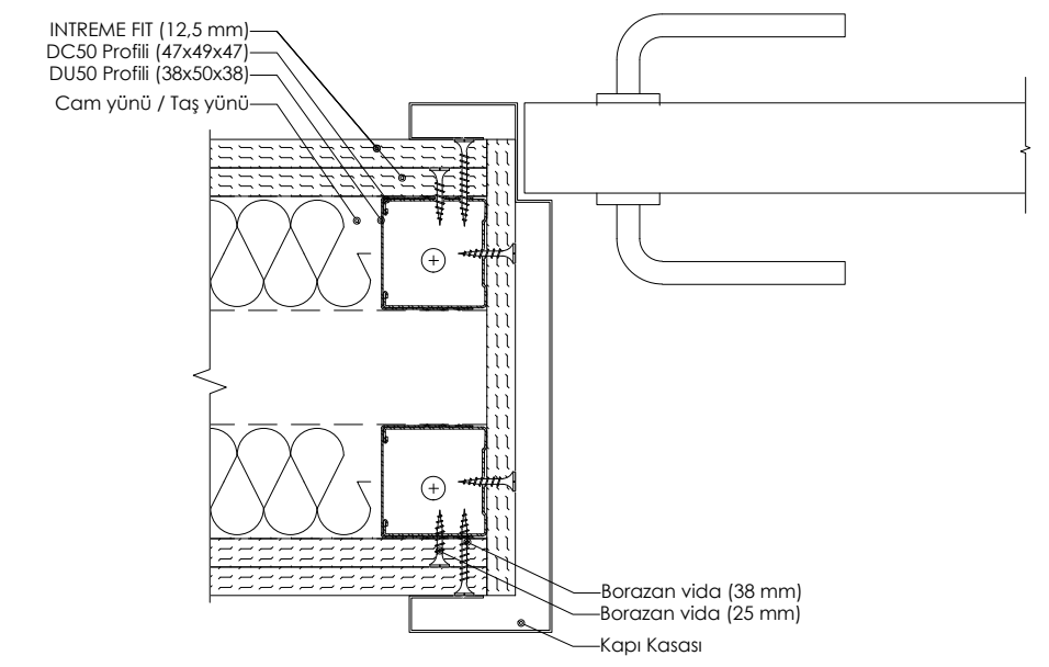
DETAY 09: ÇİFT İSKELET ÇİFT KAT INTREME FIT VİDALAMALI KAPI PLANI (BAĞLANTILI)
