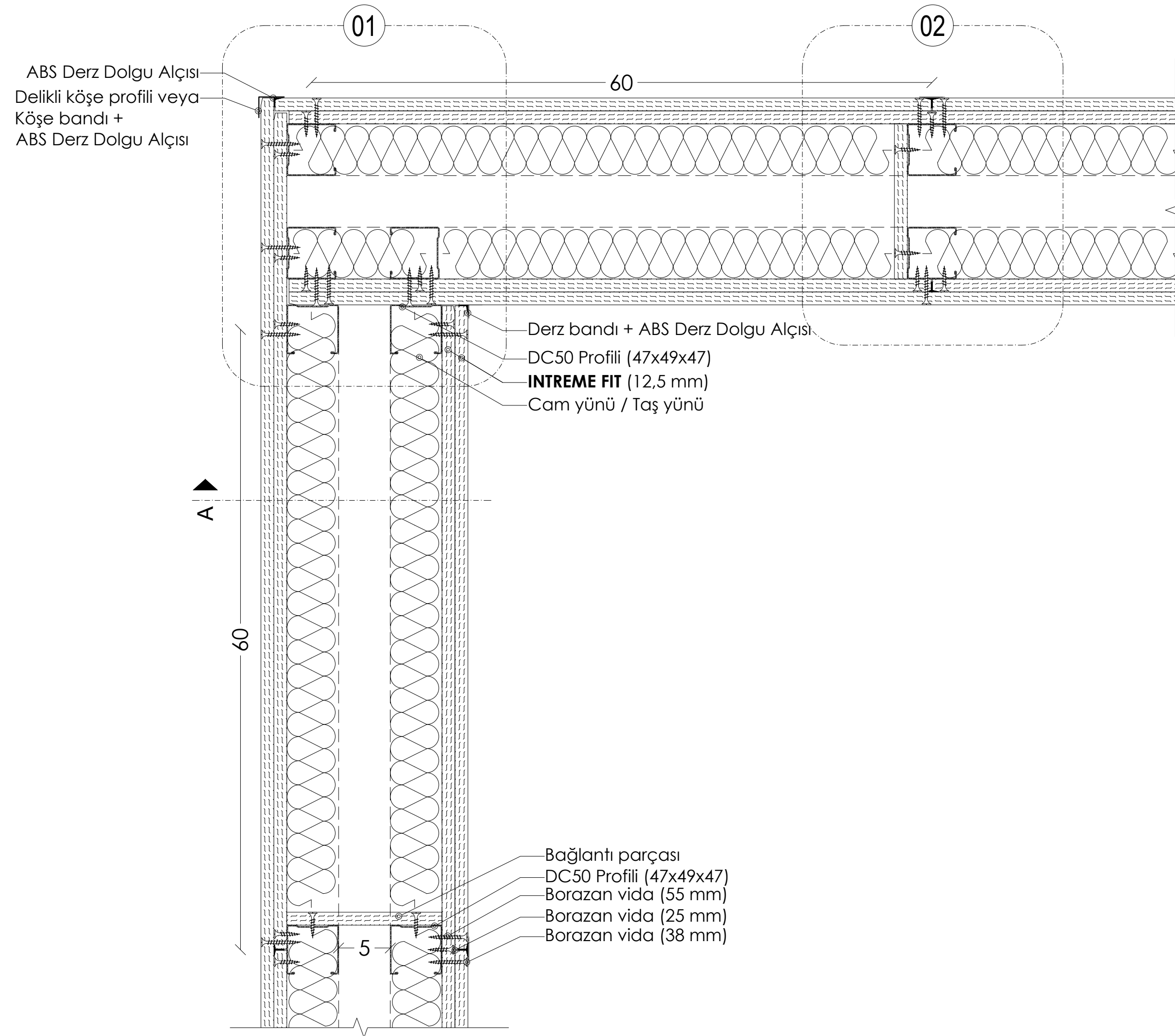
PLAN: ÇİFT İSKELET SİSTEMİ KÖŞE BİRLEŞİMİ (BAĞLANTILI)
