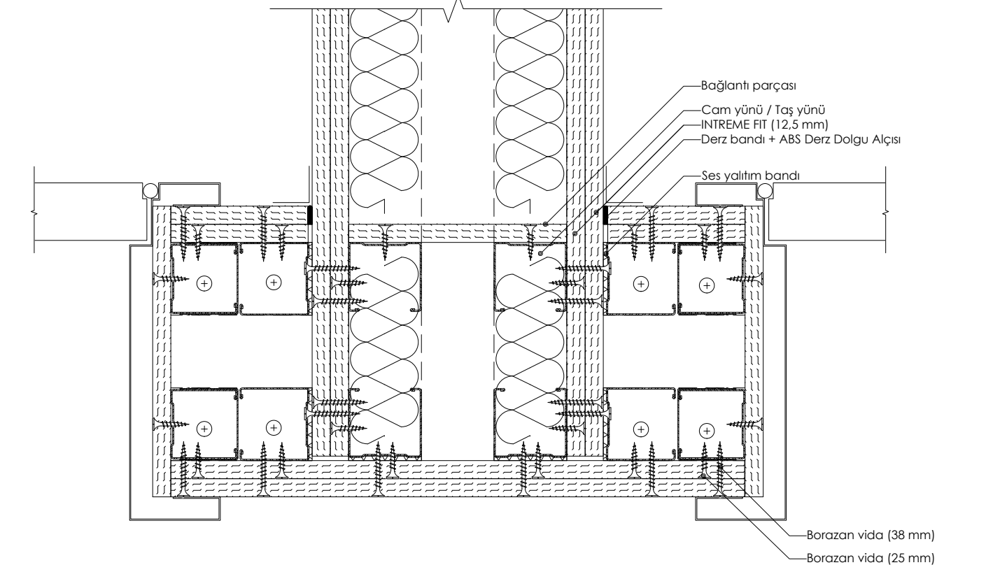
DETAY 10: ÇİFT İSKELET SİSTEMİ VİDALAMALI KAPI PLANI (BAĞLANTILI)
