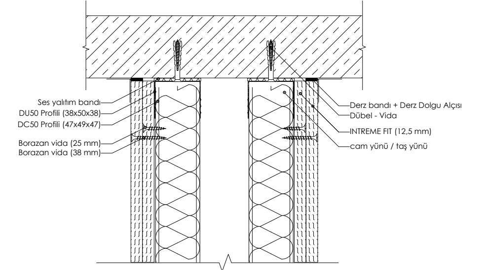
DETAY 03: ÇİFT İSKELET SİSTEMİ TAVAN BİRLEŞİM KESİTİ (BAĞLANTILI)
