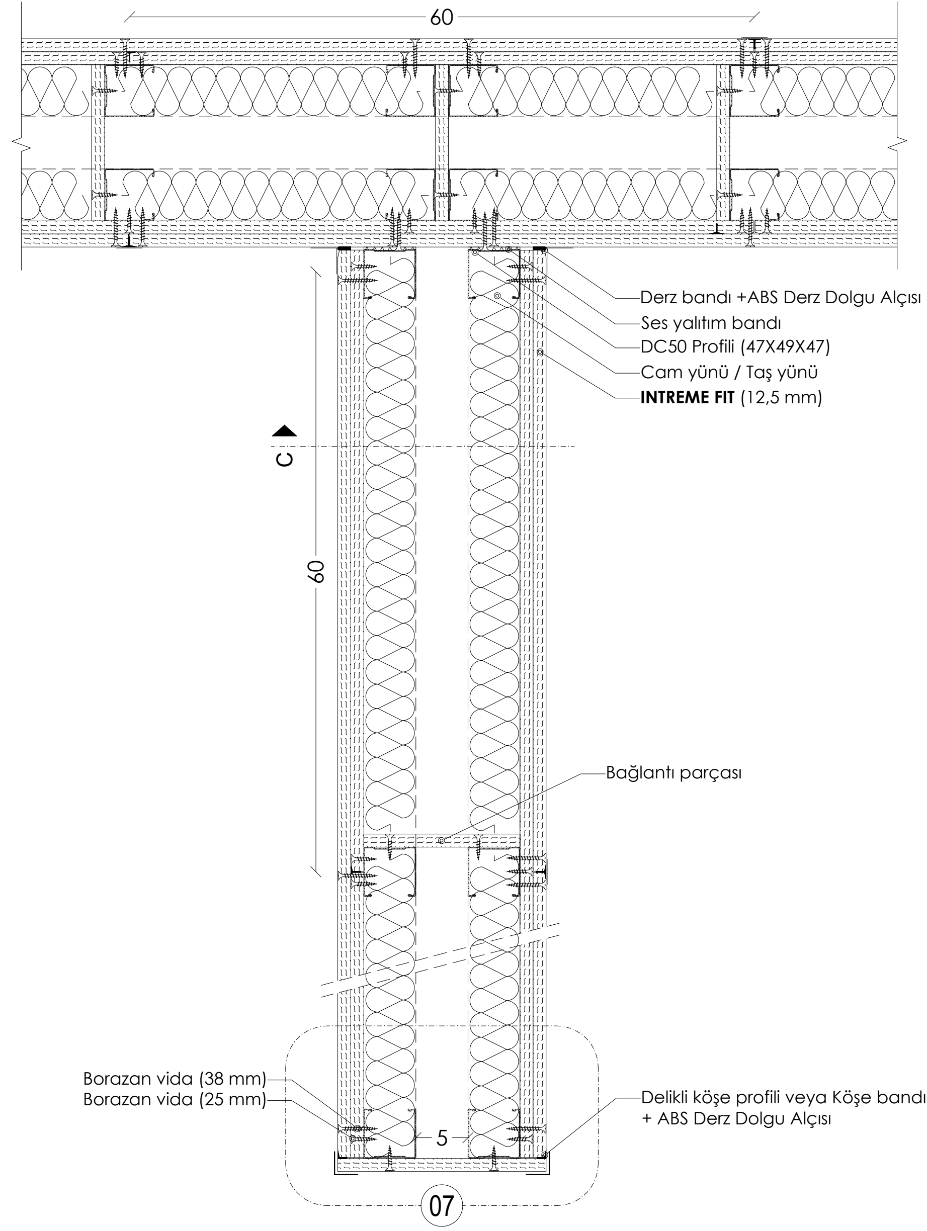
PLAN: ÇİFT İSKELET SİSTEMİ DİŞ DUVAR (BAĞLANTILI)
