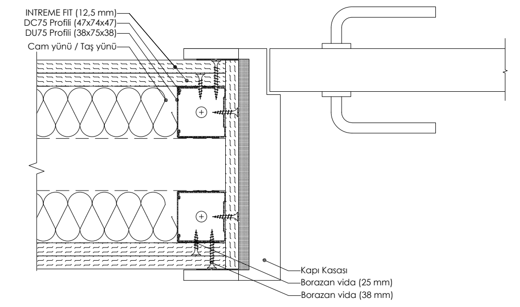
DETAY 11: ÇİFT İSKELET SİSTEMİ YAPIŞTIRMA KAPI PLANI (BAĞLANTILI)
