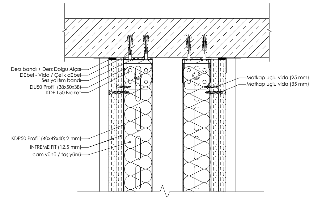
DETAY 16: ÇİFT İSKELET SİSTEMİ KAPI DESTEK PROFİLİ TAVAN BİRLEŞİM KESİTİ (BAĞLANTILI)
