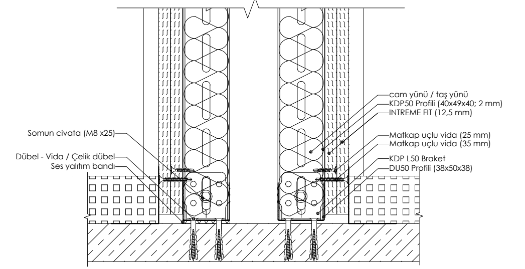
DETAY 15: ÇİFT İSKELET SİSTEMİ KAPI DESTEK PROFİLİ ZEMİN BİRLEŞİM KESİTİ (BAĞLANTILI)
