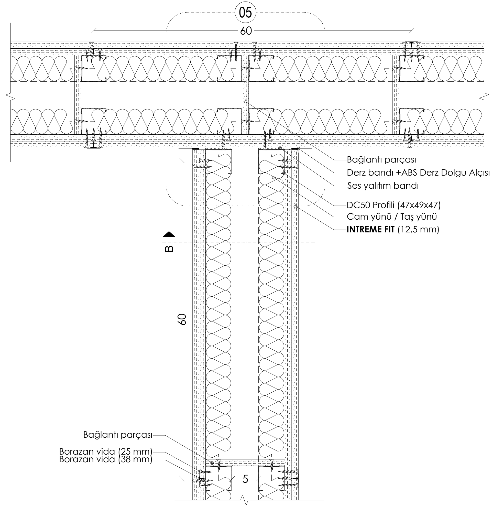
PLAN: ÇİFT İSKELET SİSTEMİ KÖŞE BİRLEŞİMİ (BAĞLANTILI)
