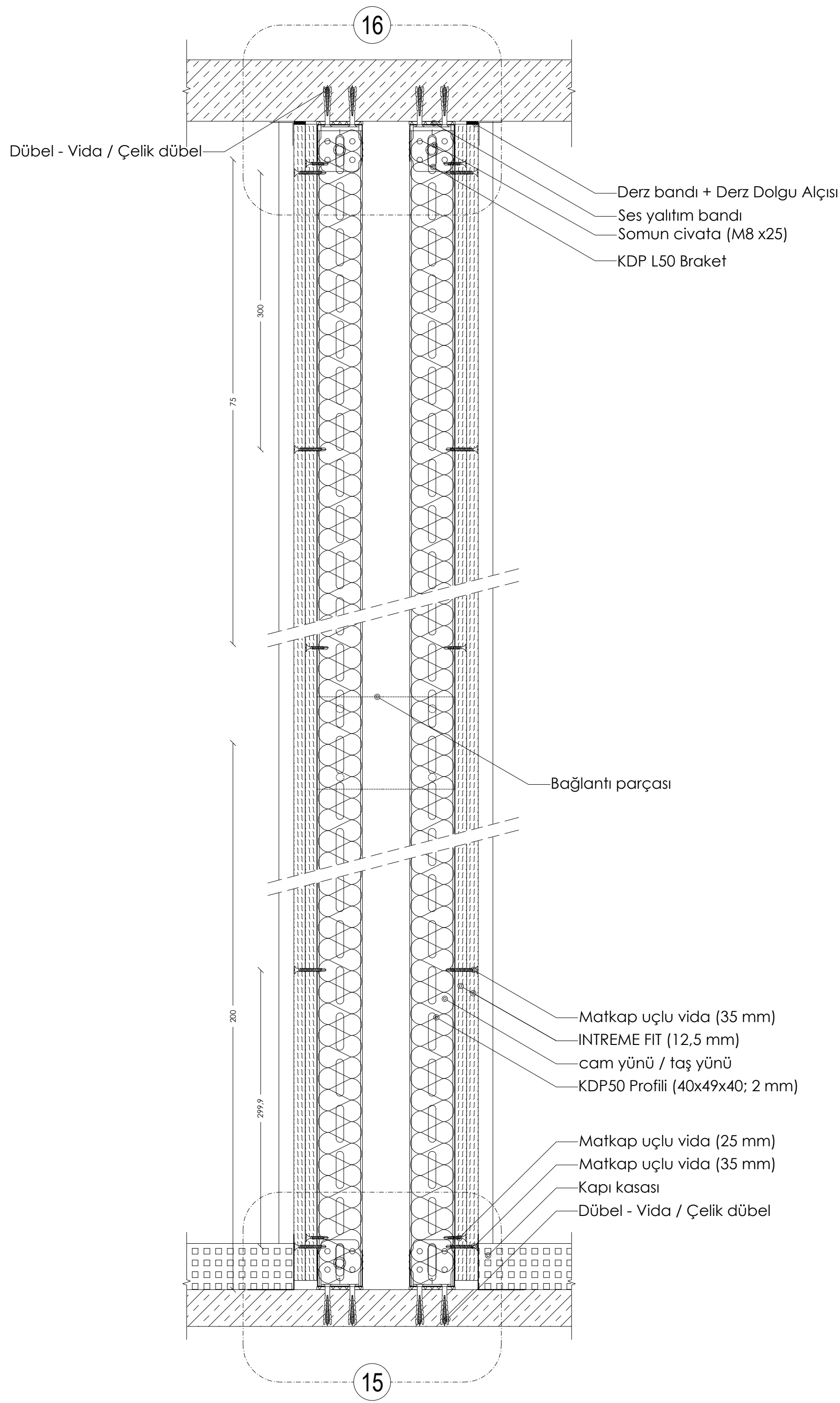
KESİT D: ÇİFT İSKELET SİSTEMİ KAPI DESTEK PROFİLİ DETAYI (BAĞLANTILI)
