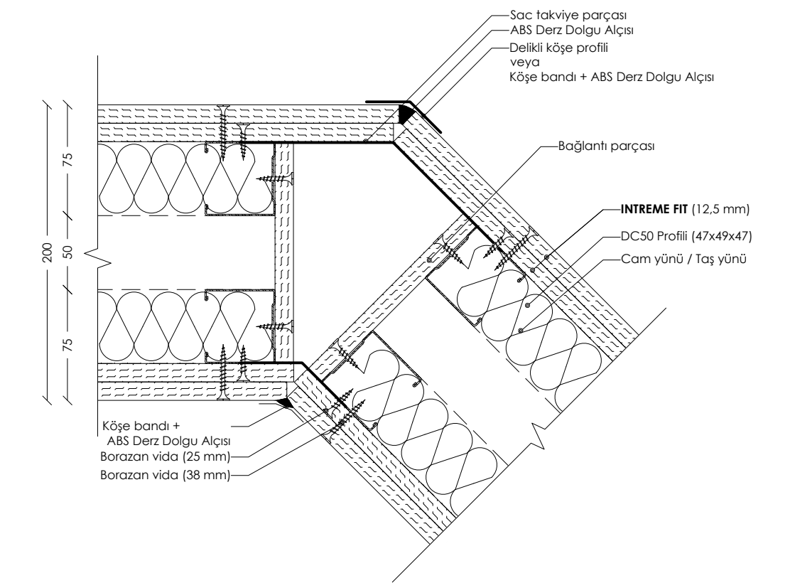
DETAY 08: ÇİFT İSKELET SİSTEMİ 135° DUVAR BİRLEŞİMİ (BAĞLANTILI)
