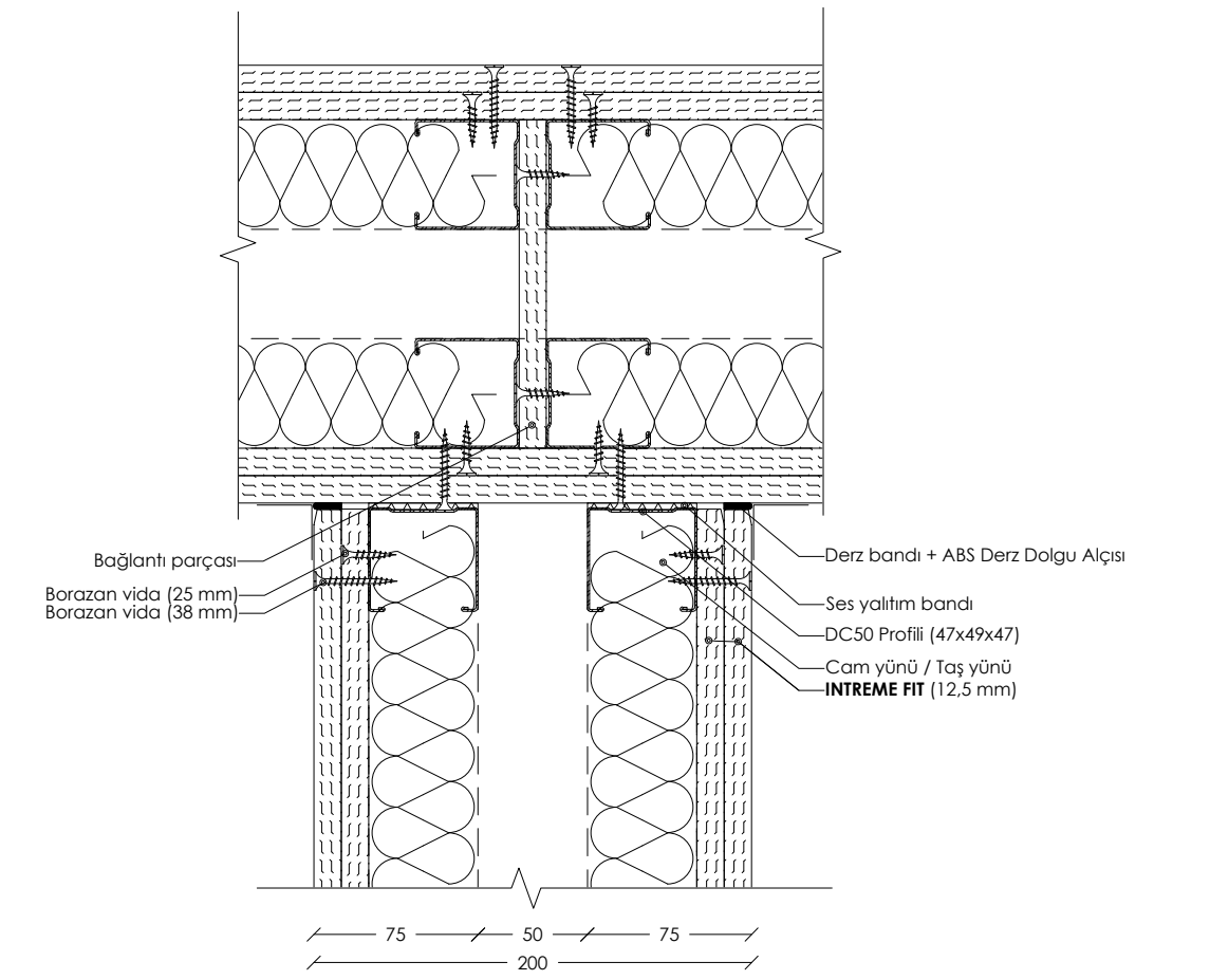
DETAY 05: ÇİFT İSKELET SİSTEMİ BİRLEŞİM PLANI (BAĞLANTILI)
