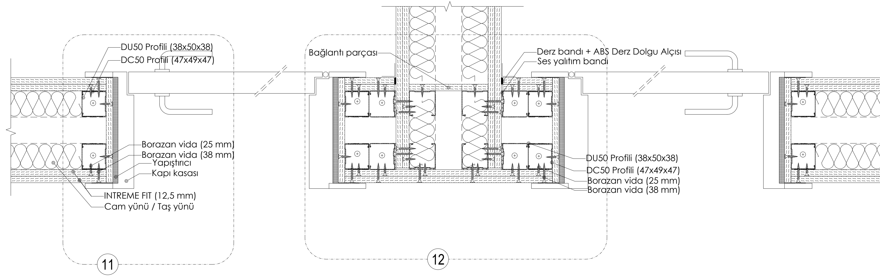
PLAN: ÇİFT İSKELET SİSTEMİ YAPIŞTIRMA KAPI DETAYI (BAĞLANTILI)
