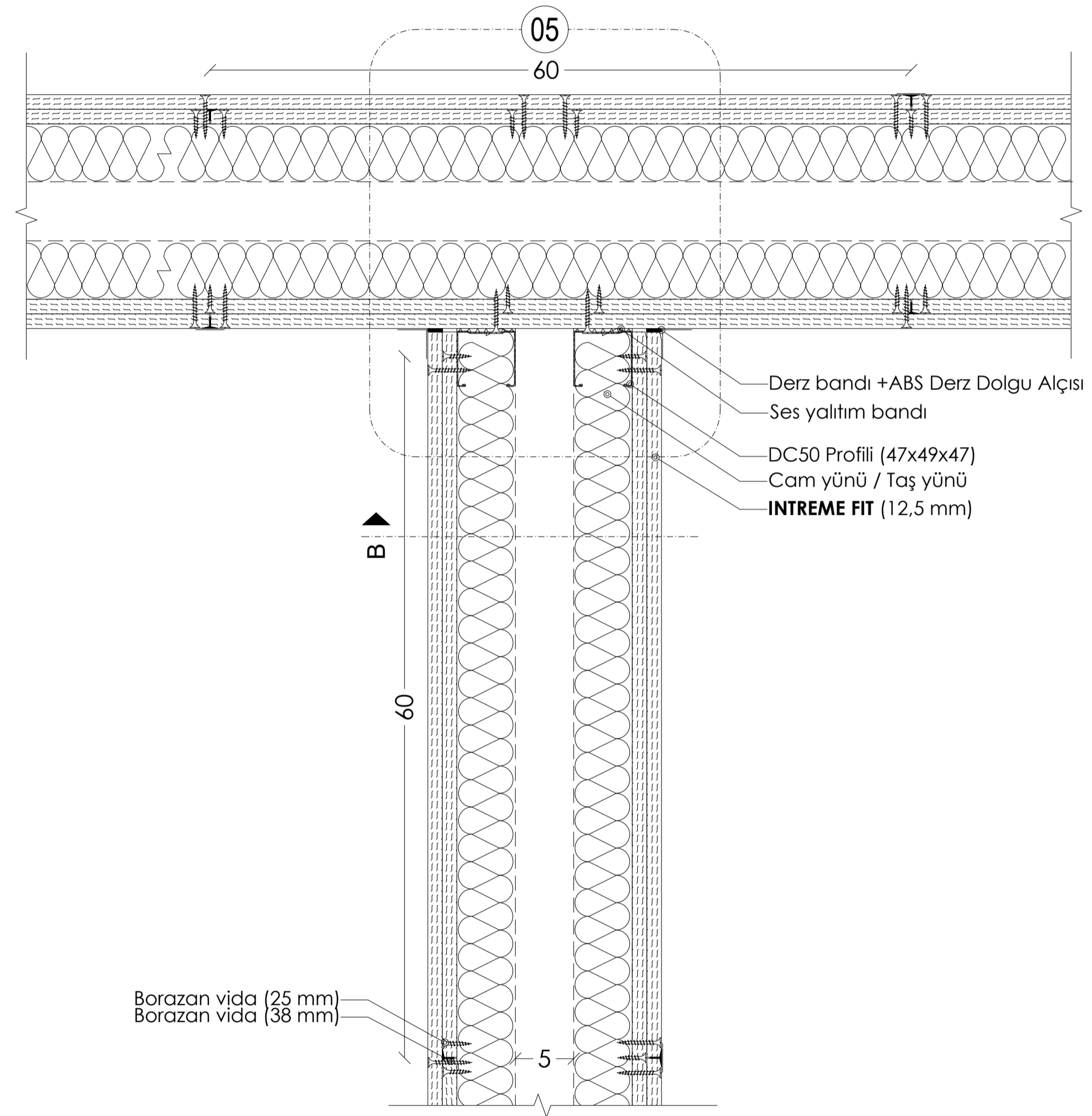
PLAN: ÇİFT İSKELET SİSTEMİ KÖŞE BİRLEŞİMİ
