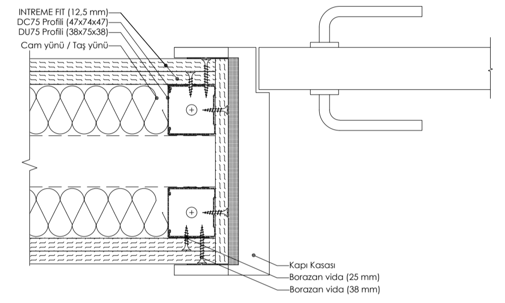
DETAY 11: ÇİFT İSKELET SİSTEMİ YAPIŞTIRMA KAPI PLANI (BAĞLANTILI)
