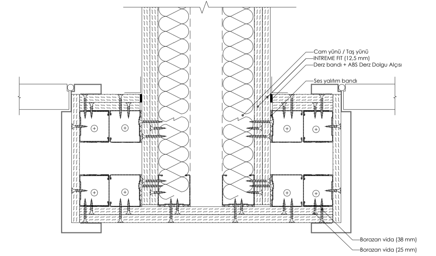
DETAY 10: ÇİFT İSKELET SİSTEMİ VİDALAMALI KAPI PLANI
