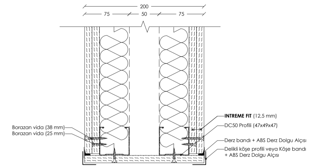
DETAY 07: ÇİFT İSKELET SİSTEMİ DİŞ DUVAR PLANI
