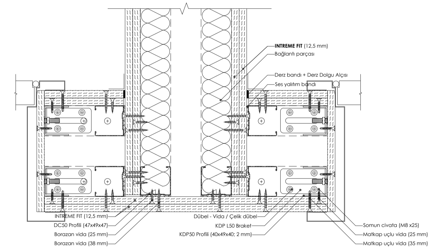
DETAY 14: ÇİFT İSKELET SİSTEMİ KAPI DESTEK PROFİLİ DETAYI
