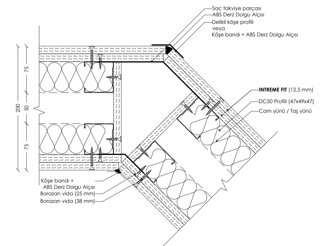
DETAY 08: ÇİFT İSKELET SİSTEMİ 135° DUVAR BİRLEŞİMİ
