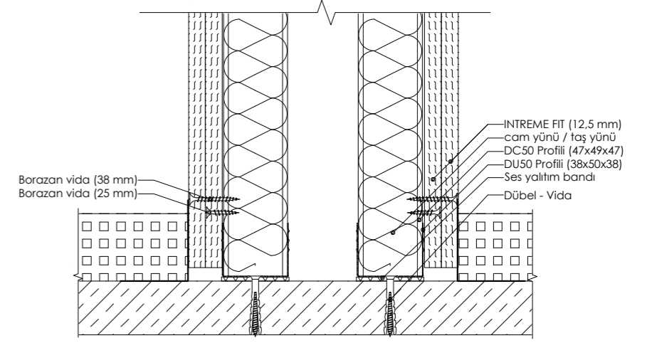
DETAY 04: ÇİFT İSKELET SİSTEMİ ZEMİN BİRLEŞİM KESİTİ
