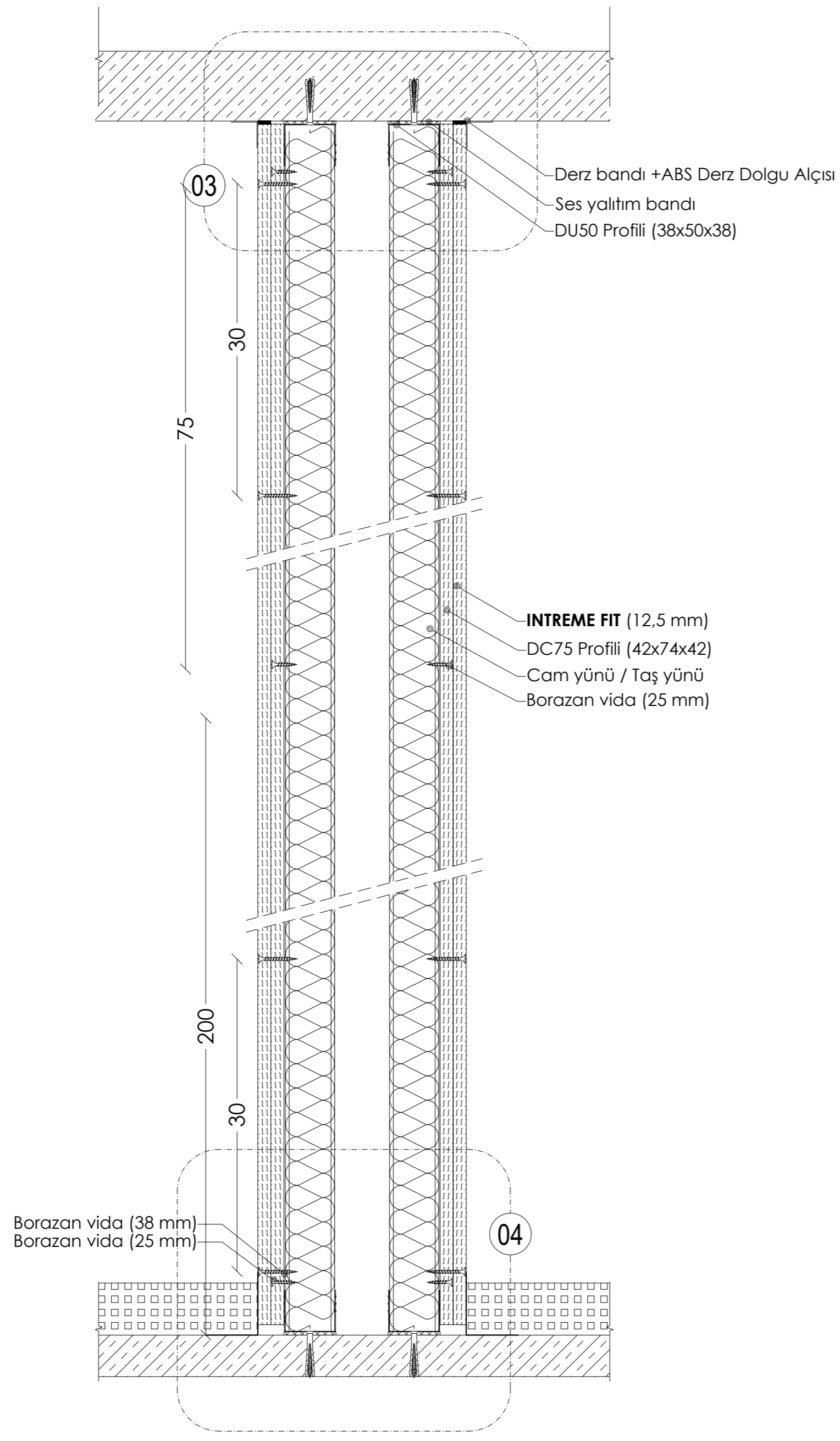
KESİT A: ÇİFT İSKELET SİSTEMİ
