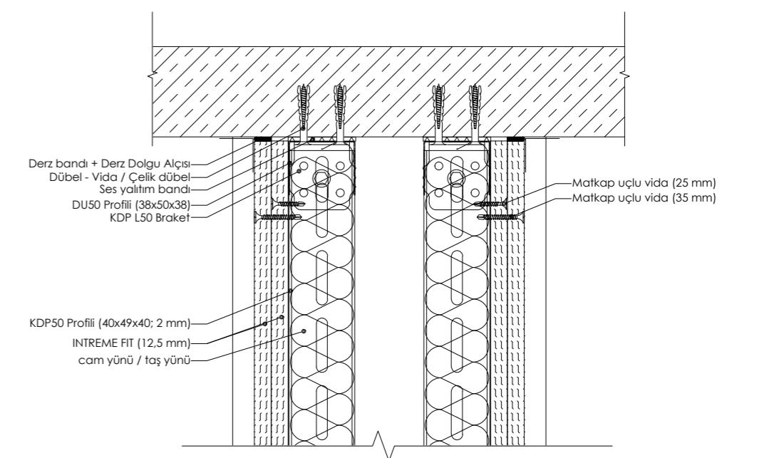
DETAY 16: ÇİFT İSKELET SİSTEMİ KAPI DESTEK PROFİLİ TAVAN BİRLEŞİM KESİTİ
