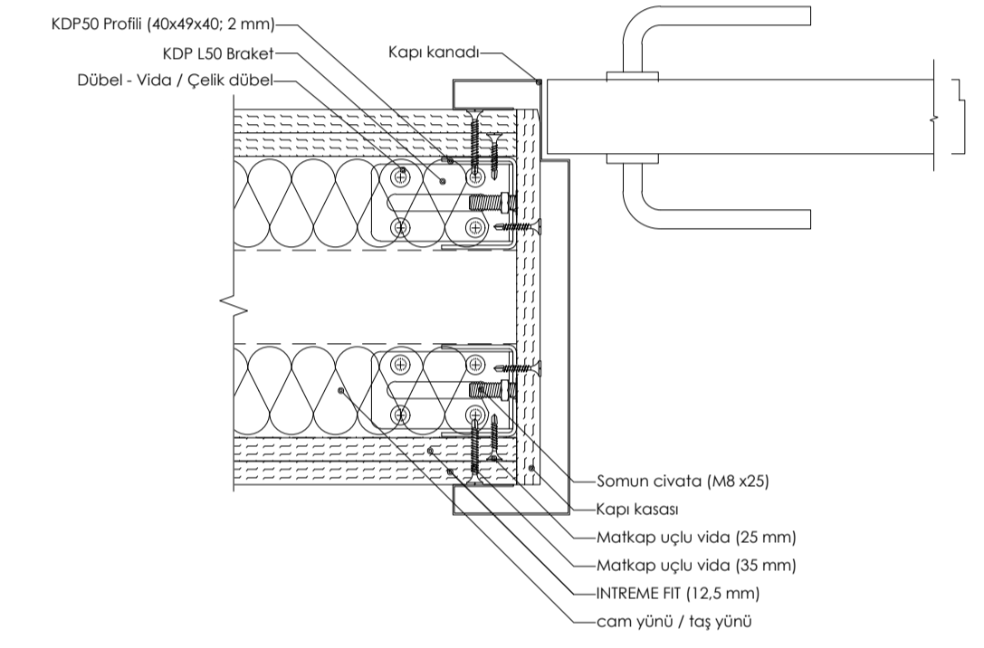
DETAY 13: ÇİFT İSKELET SİSTEMİ KAPI DESTEK PROFİLİ DETAYI
