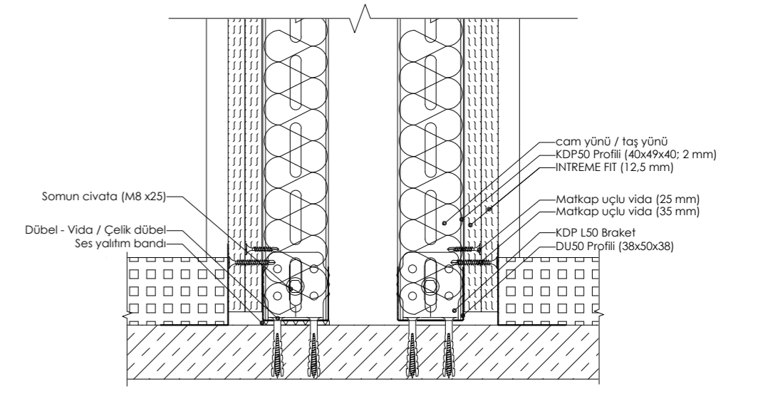
DETAY 15: ÇİFT İSKELET SİSTEMİ KAPI DESTEK PROFİLİ ZEMİN BİRLEŞİM KESİTİ
