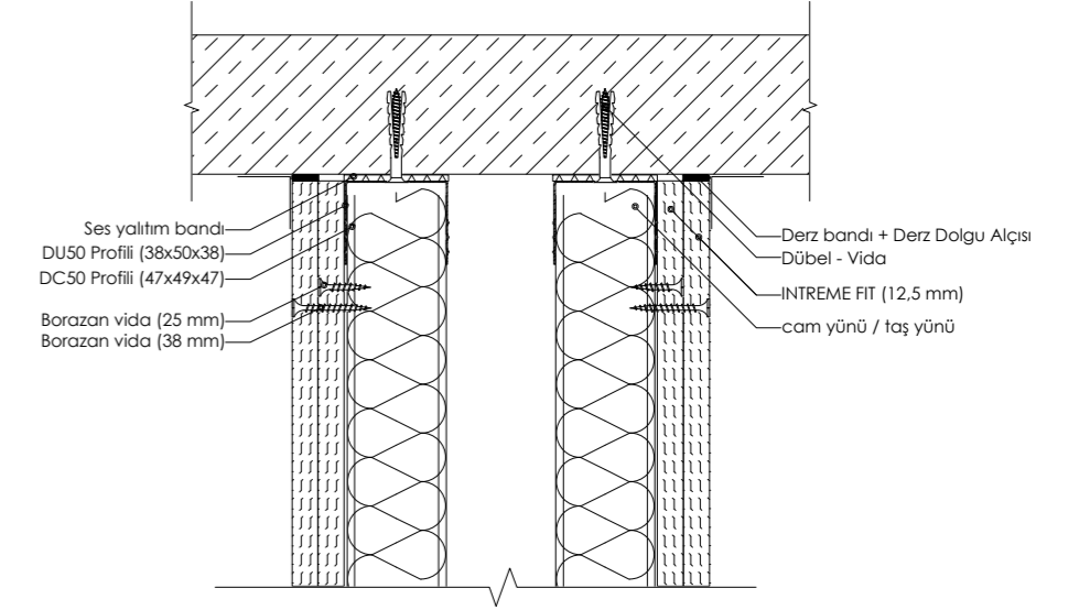
DETAY 03: ÇİFT İSKELET SİSTEMİ TAVAN BİRLEŞİM KESİTİ
