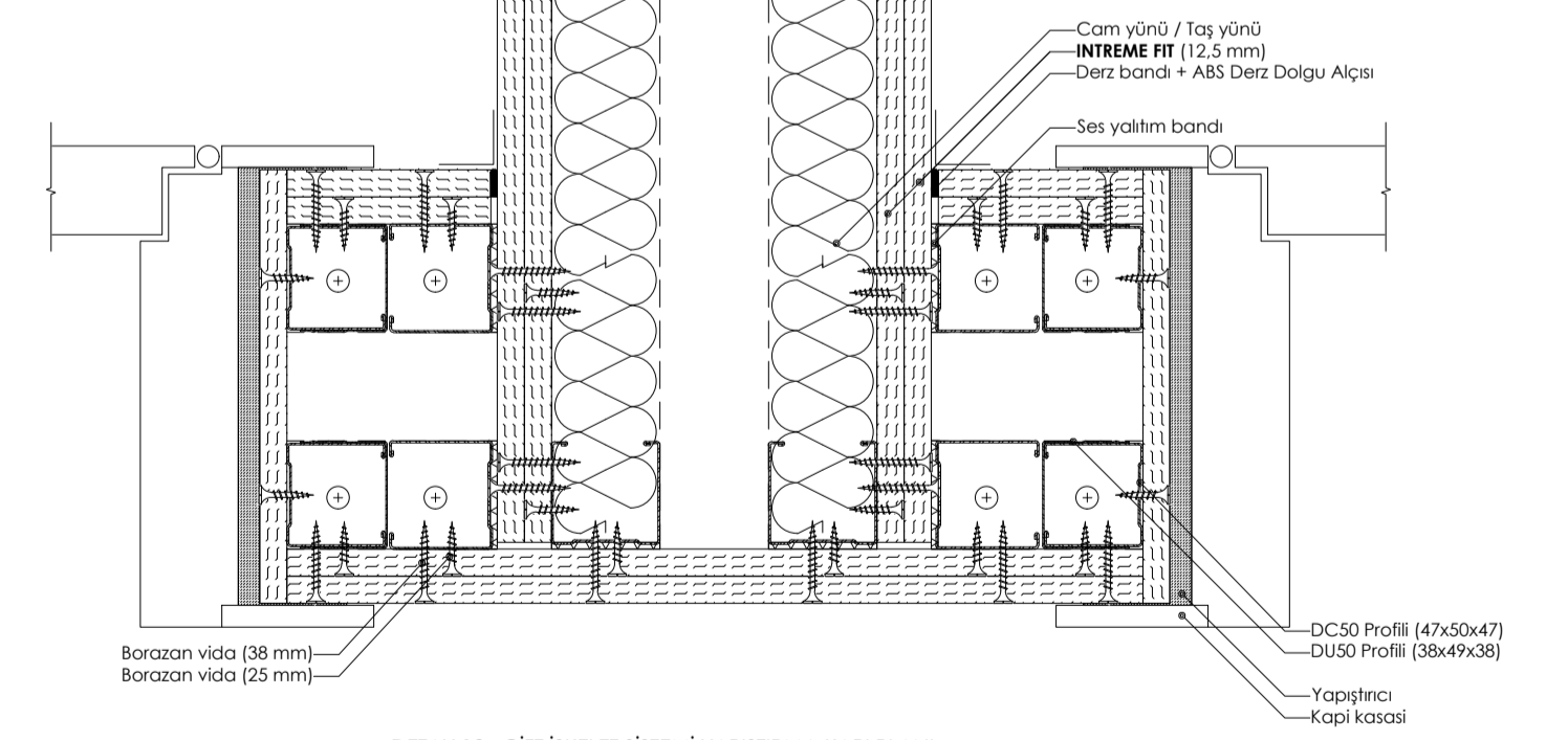
DETAY 12: ÇİFT İSKELET SİSTEMİ YAPIŞTIRMA KAPI PLANI
