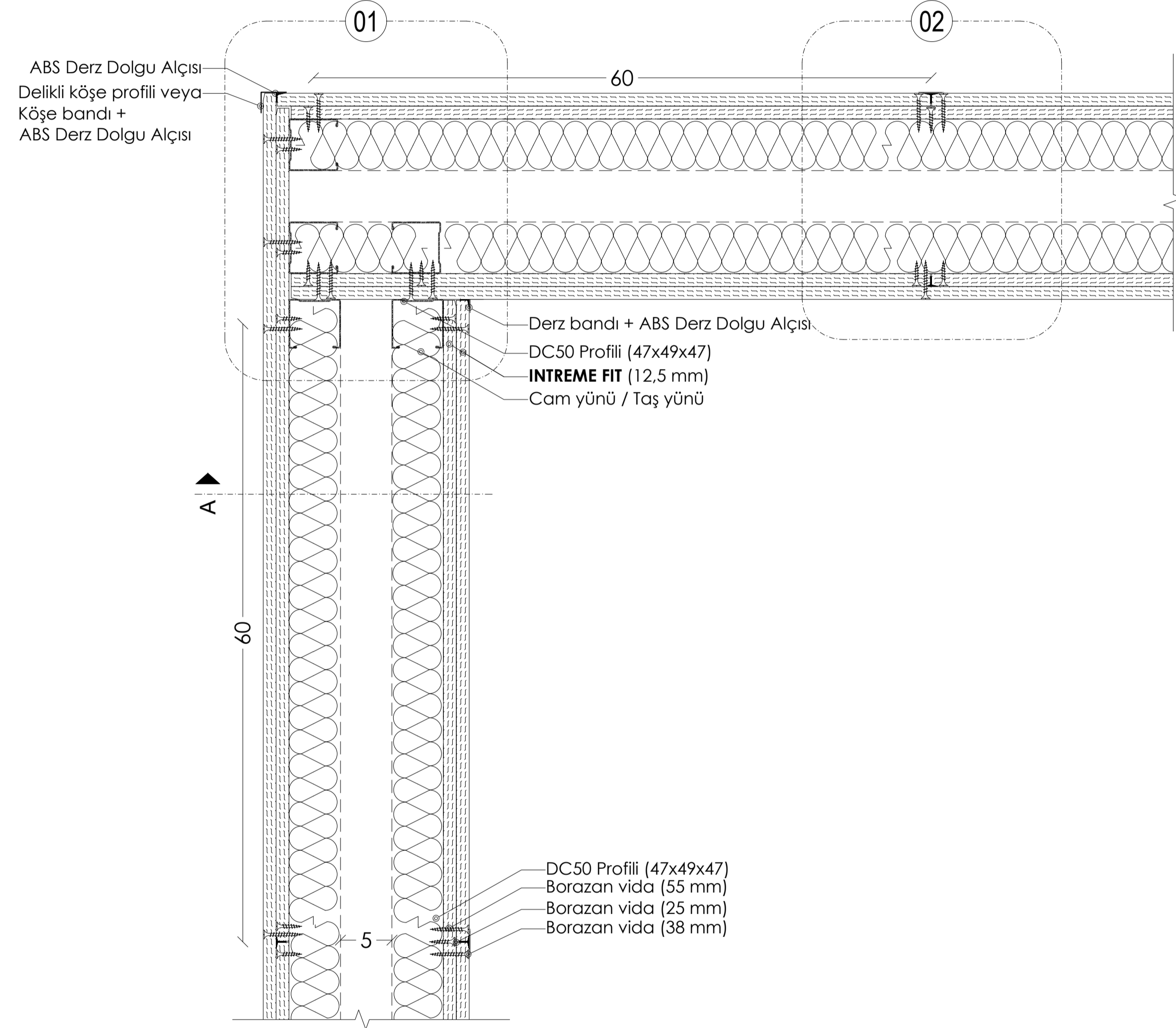
PLAN: ÇİFT İSKELET SİSTEMİ KÖŞE BİRLEŞİMİ
