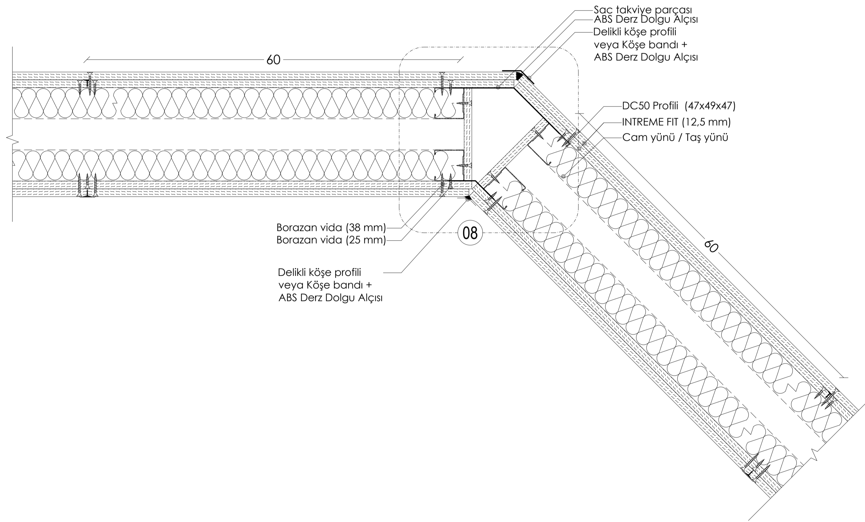
PLAN: ÇİFT İSKELET SİSTEMİ 135° DUVAR BİRLEŞİMİ
