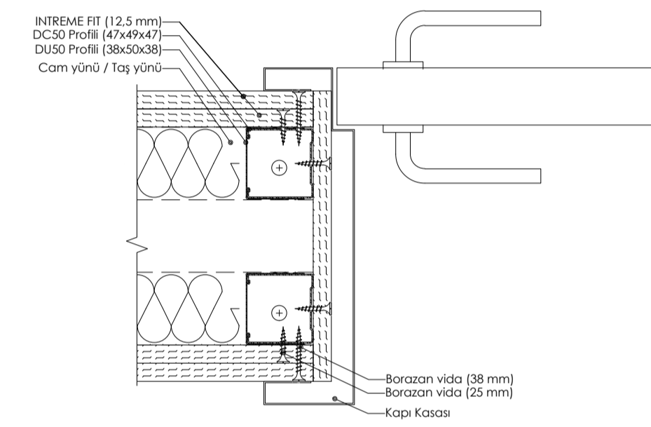
DETAY 09: ÇİFT İSKELET ÇİFT KAT INTREME FIT VİDALAMALI KAPI PLANI
